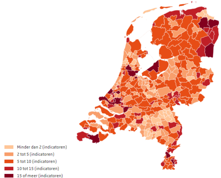
Figuur 3: Kaartbeeld aantal indicatoren (Hier & Nu) waarvoor een gemeente behoort tot de bovenste (links) of onderste (rechts) kwart van de ranglijst van gemeenten (Bron: Regionale Monitor CBS )
