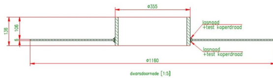
Figuur 8 - indicatieve weergave doorvoer.
