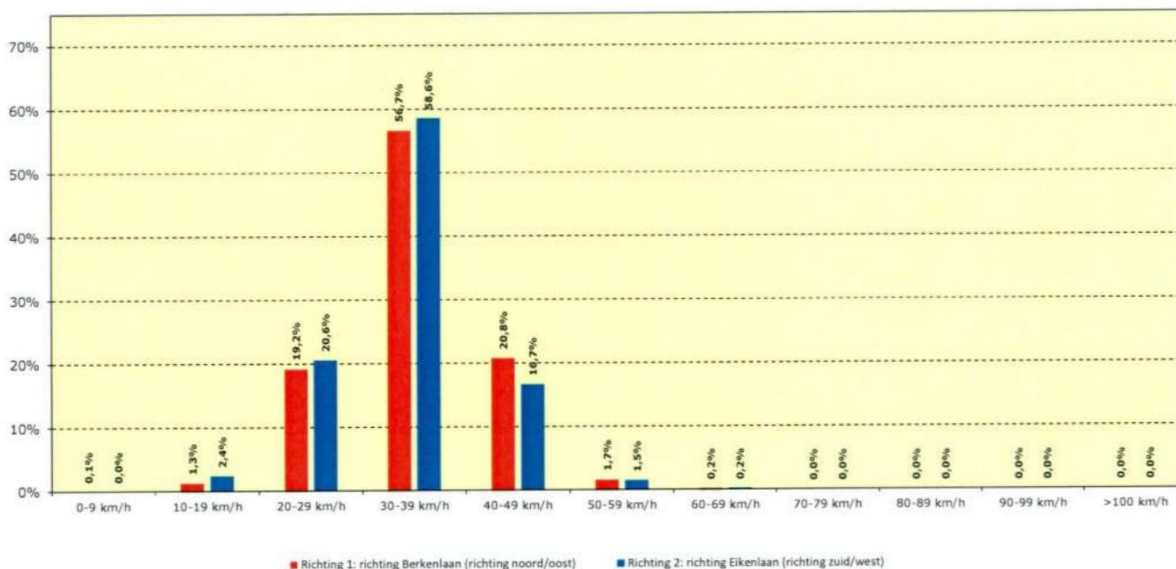
Verdeling snelheden per richting (categorie 2 + 3)
