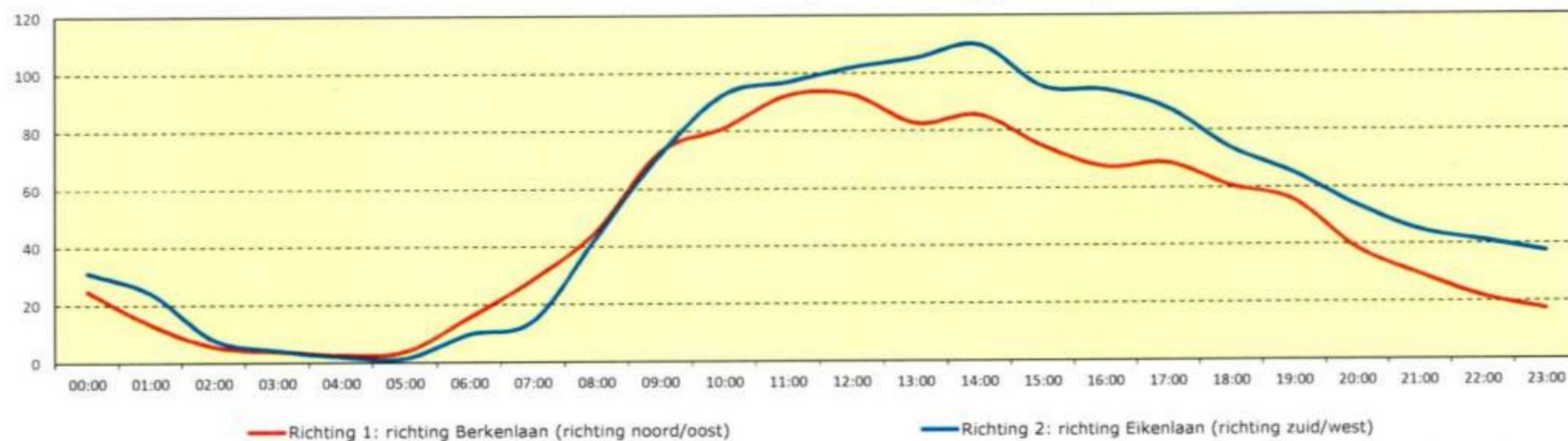
Gemiddelde uurintensiteiten per weekenddag (cat. 2+3)
