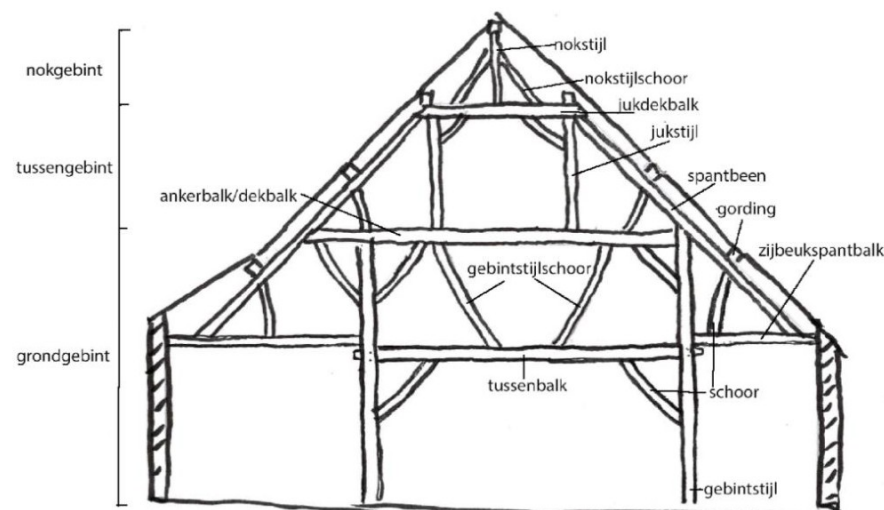
Afb. 141 Schematische weergave van de houtconstructie van de Beijlshof.
