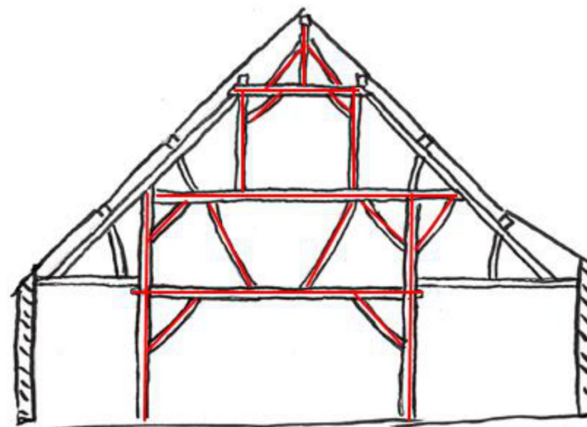
Afb. 218 Gebint van de schuur. In rood de constructie van de oude vakwerkschuur.
