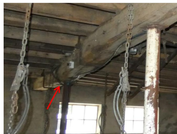
Afb. 49 De moerbalk in de stal, waar aan de zuidzijde een klein pengat zichtbaar is (stijl van de voormalige voergang).
