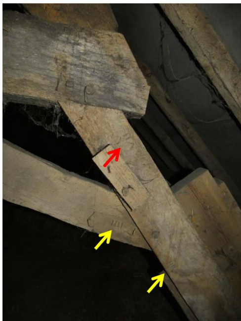
Afb. 55 Spant vier, zuidzijde. Zowel nummering IIII (geel) als VII (rood)
