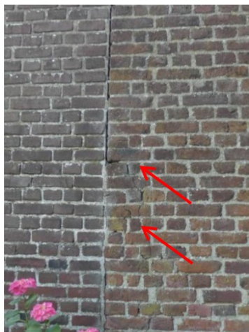
Afb. 220 Kruisverband met klezoren bij de schuur.
