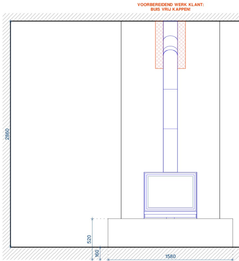
VOORAANZICHT
