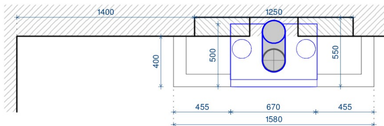
BOVENAANZICHT HAARD
