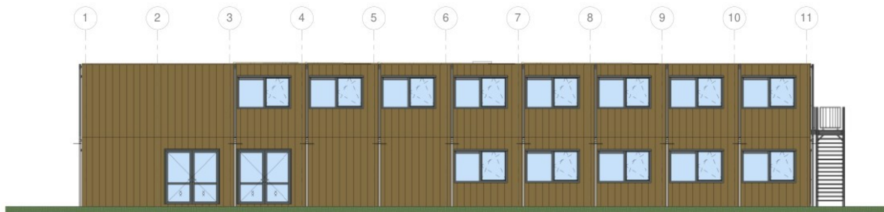
Voorgevel schaal 1 : 100
