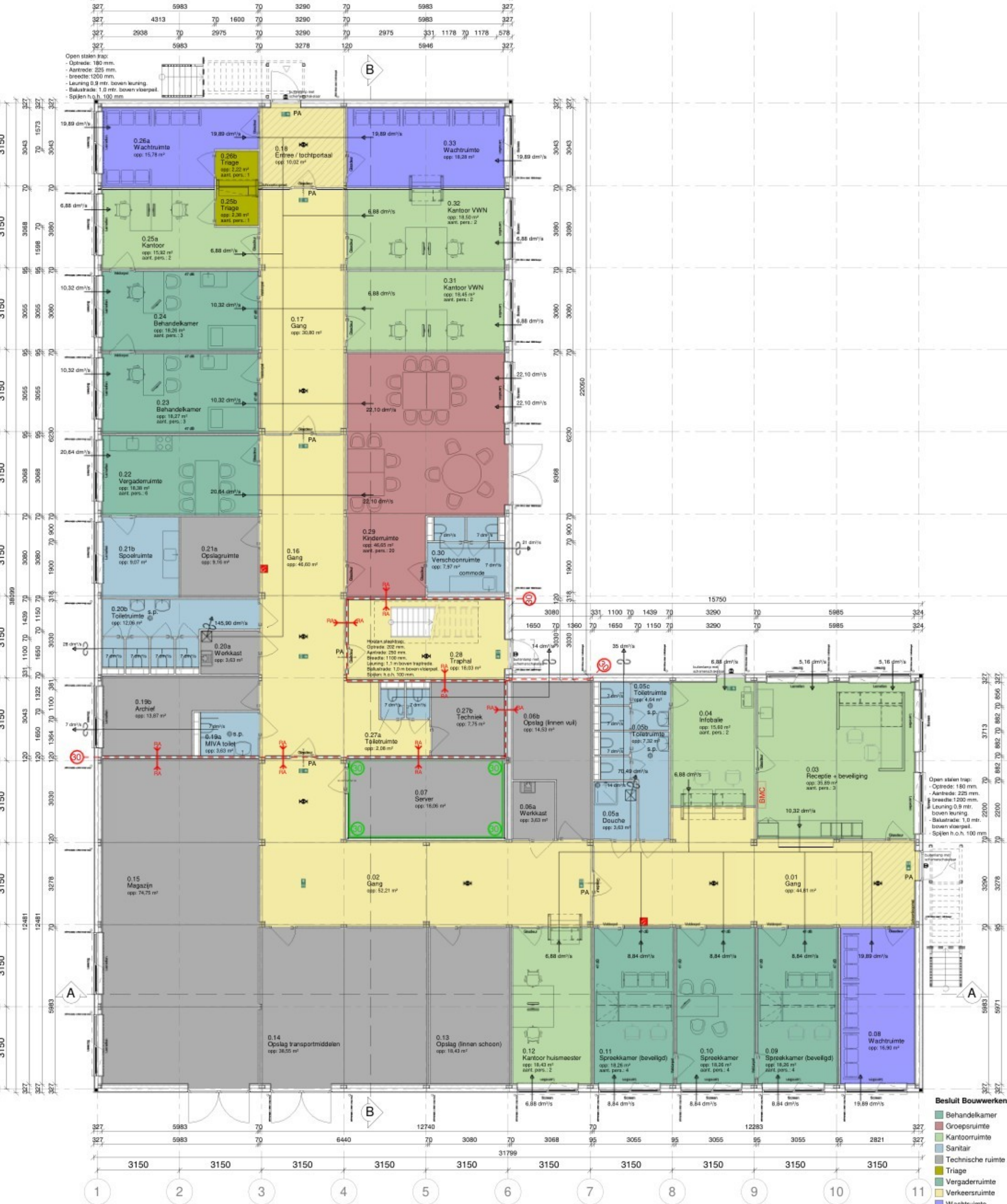
Begane grond schaal 1 : 100
