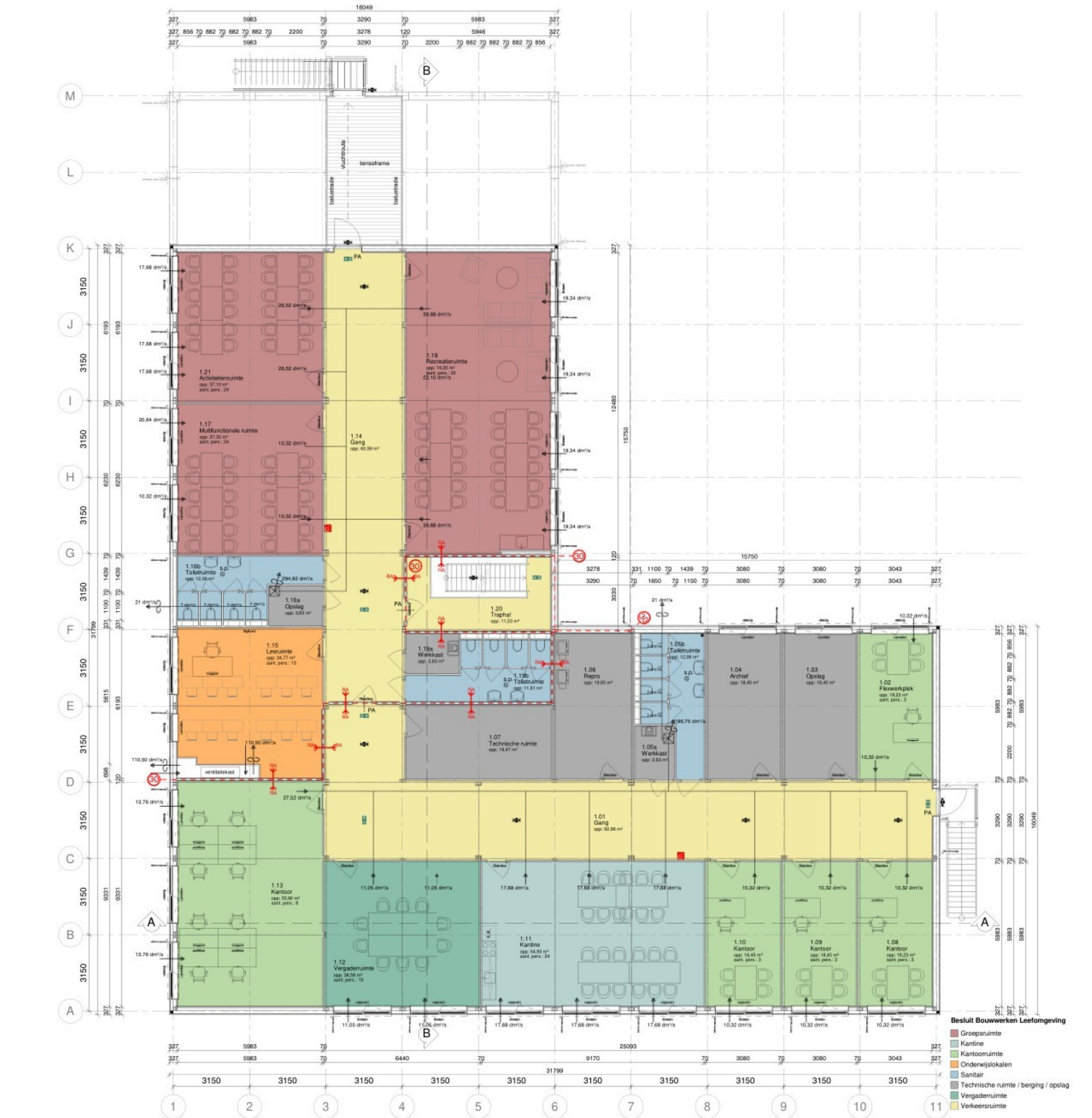
Verdieping schaal 1 : 100
