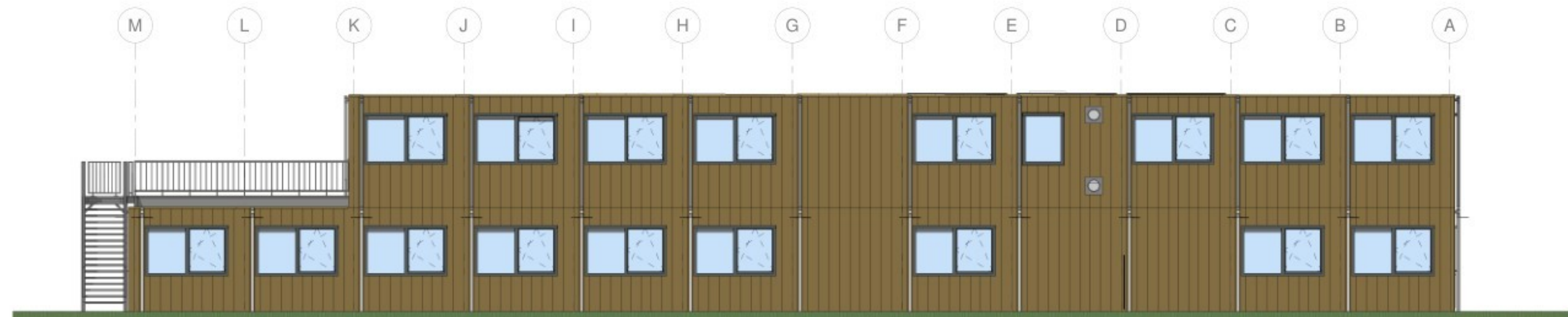
Linker zijgevel schaal 1 : 100
