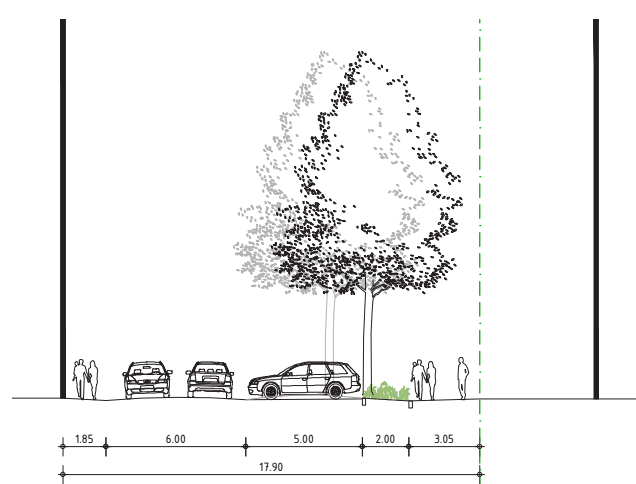
profiel BB
