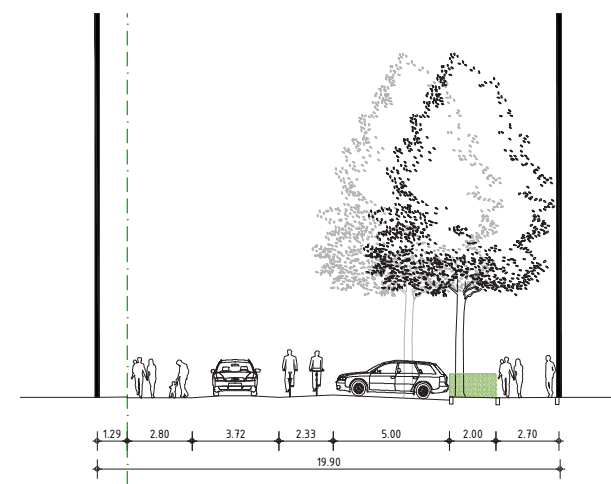
profiel CC
