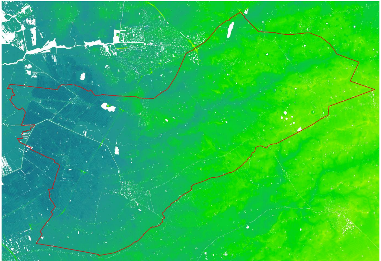
Weergave van de Actuele Hoogtekaart Nederland (AHN). Rechts de uitlopers van het Fries-Drents plateau. De beek, in het blauw, kronkelt door deze hoger gelegen delen heen. Links het dieper gelegen lage midden. De blauwe kleur toont dat het landschap hier een stuk lager ligt. Bron: AHN Nederland.
