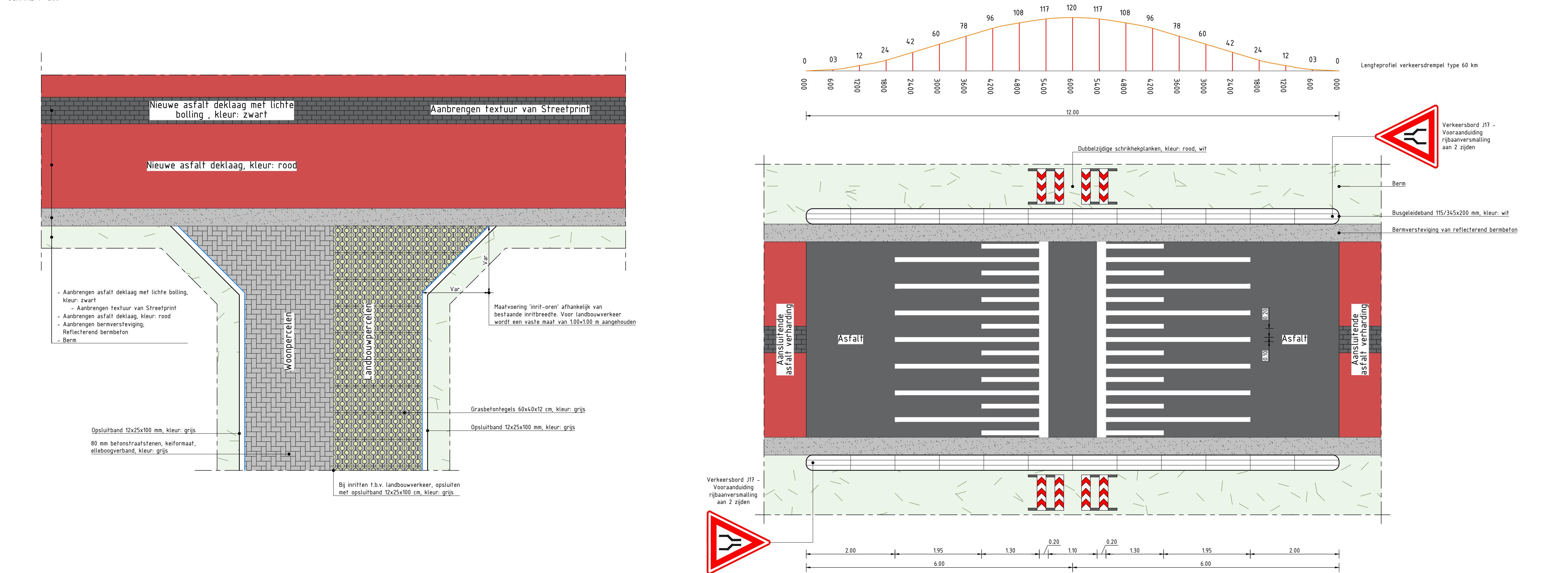
DETAIL 01: Nieuwe inritconstructie woon- en landbouwpercelen SCHAAL 1:50
