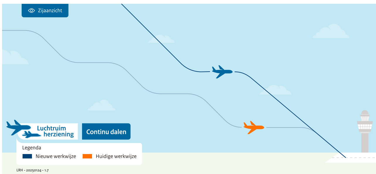
Figuur 2: Zijaanzicht met huidige werkwijze van trapsgewijs naderen via vectoren en nieuwe werkwijze middels continu dalen over vaste naderingsroute. Schets is indicatief en niet op schaal.
