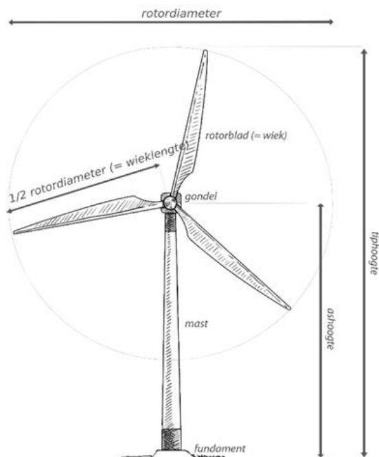
Figuur 3-3. Begrippen windturbines.
