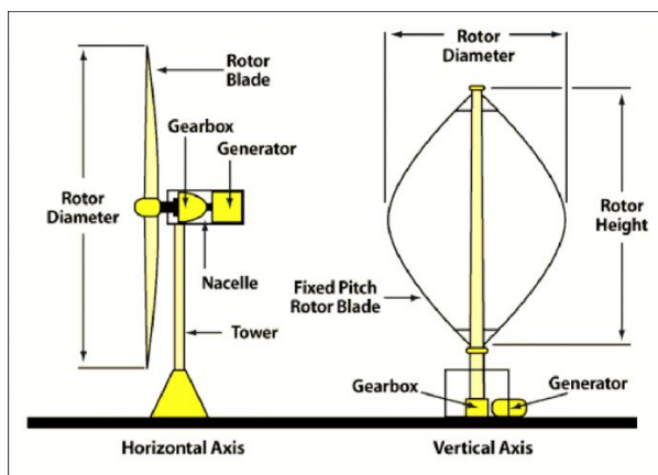
Figuur 3-1. Verschil HAWT (links) en VAWT (rechts) (Ba Alawi, 2018).
