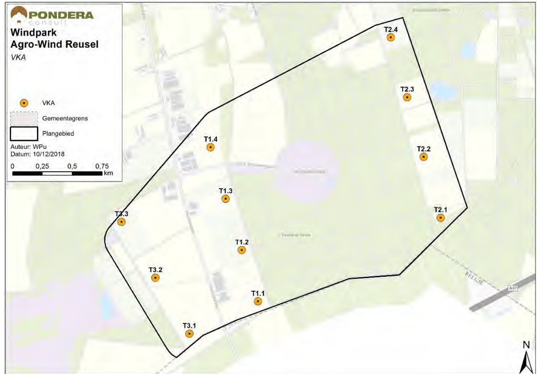
Figuur 4.3 Voorkeursalternatief
