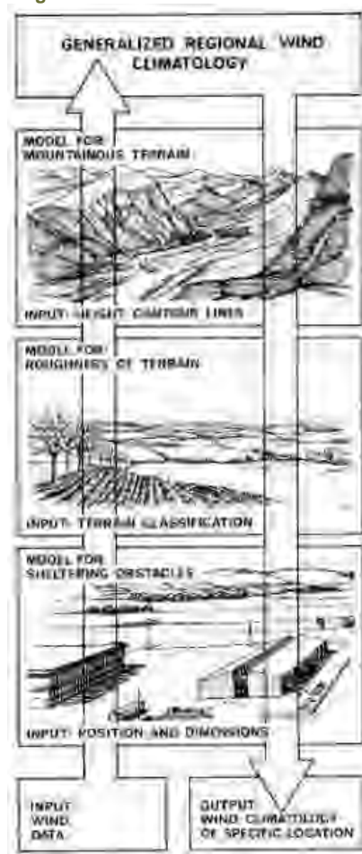
Figuur 2.2 Windatlasmethode
