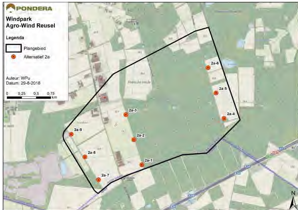
Figuur 1.7 Opstelling alternatief 2a
