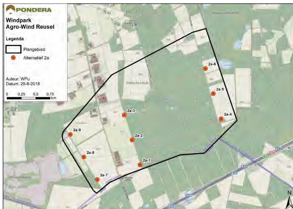
Figuur 4.2 Opstelling alternatief 2a
