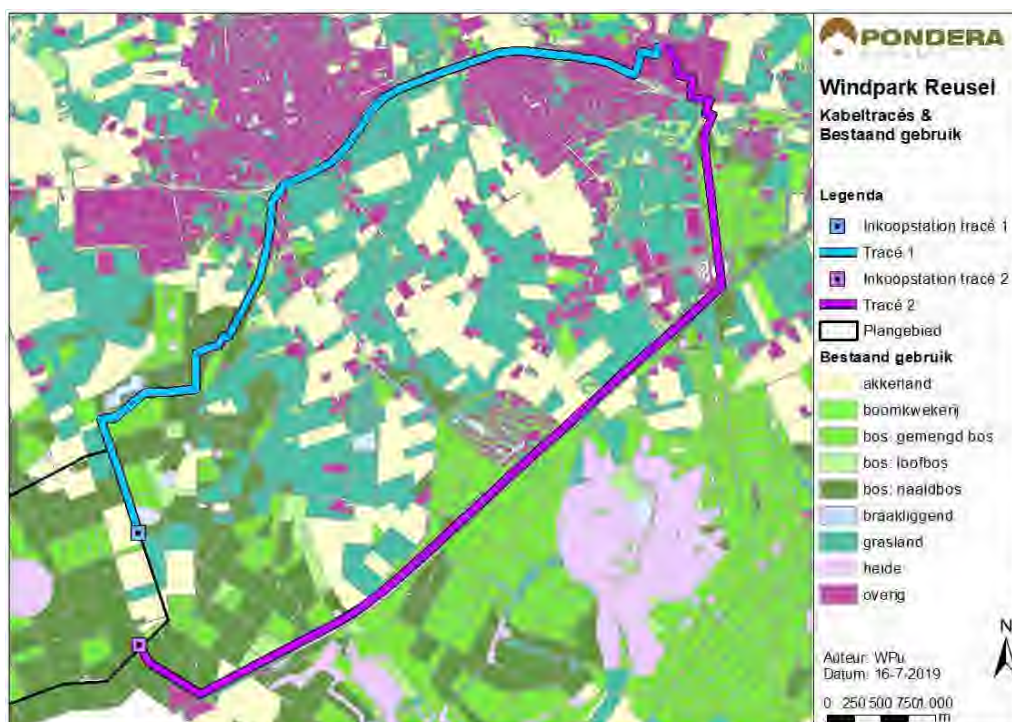
Figuur 14.4 Kabeltracés en bestaand gebruik
