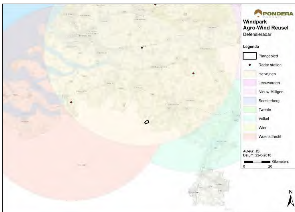
Figuur 14.3 Defensieradar
