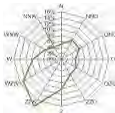
Figuur 3.2 Distributie windrichtingen bij windsnelheid > 2 m/s
