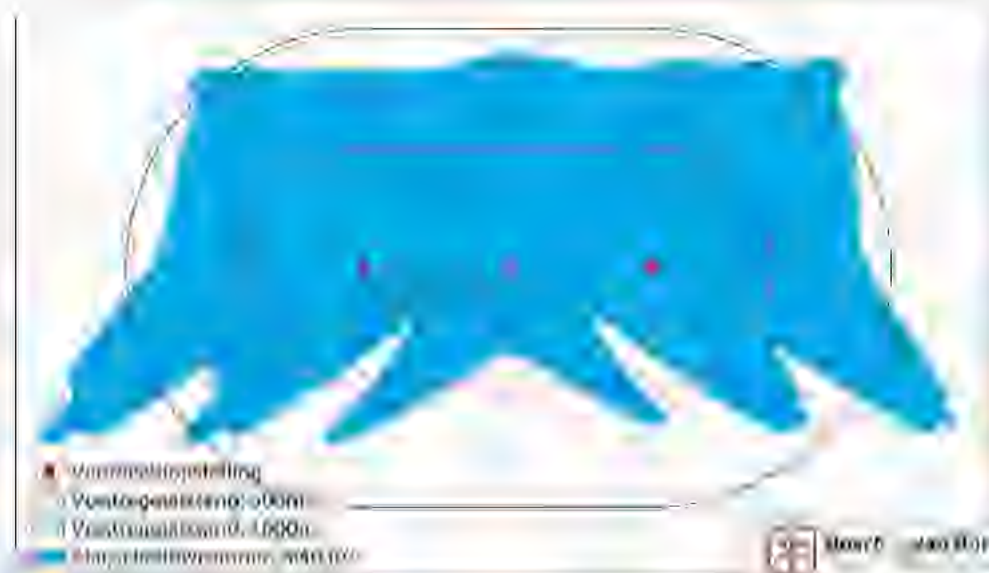
Figuur 15 Slagschaduwberekening van een voorbeeldopstelling. Binnen het blauwe vlak is de verwachte slagschaduw meer dan 5:40 uur per jaar en zou er dus een stilstandvoorziening moeten worden getroffen voor binnen het vlak liggende woningen.
