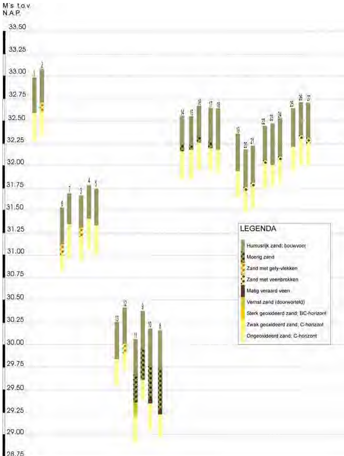
Figuur 4: Boorprofielen van de boringen 1 tot en met 27
