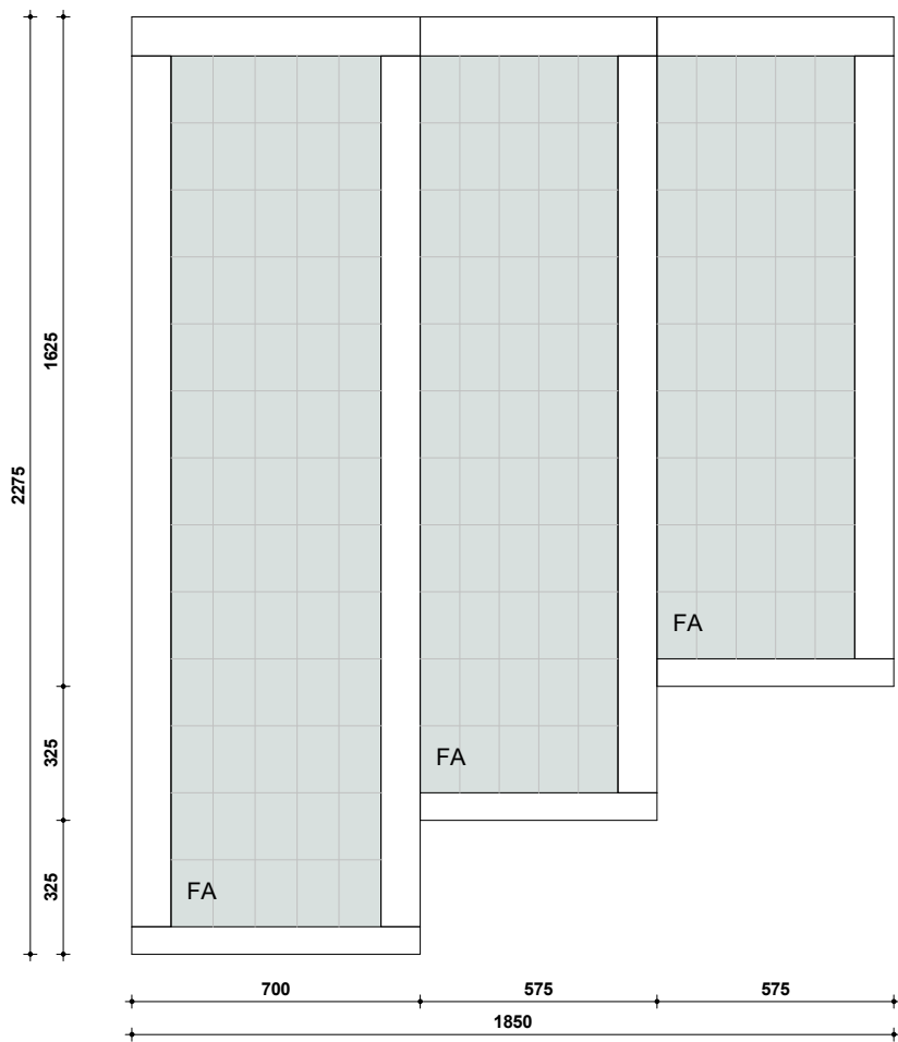
merk U - bestaand kozijn
