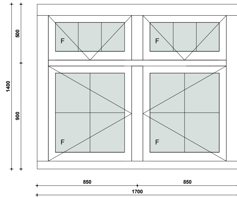
merk E - bestand kozijn
