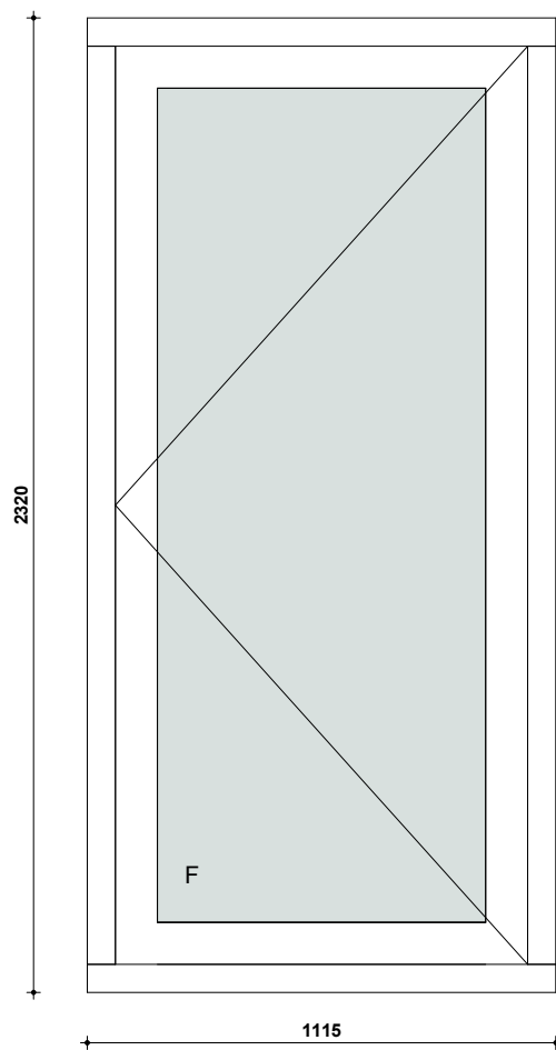
merk D - nieuw kozijn
