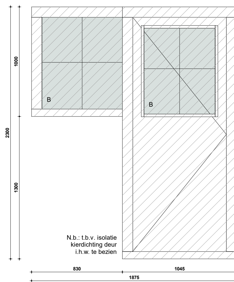
merk G - ongewijzigd
