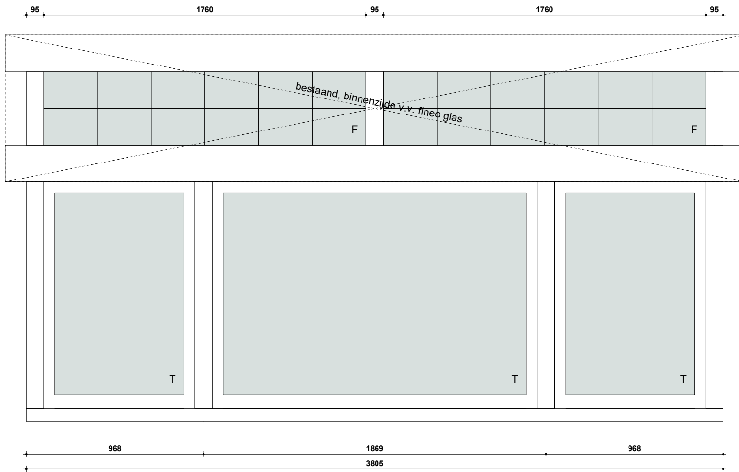
merk A - onderzijde nieuw
