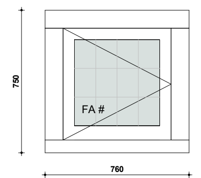
merk J - bestand kozijn
