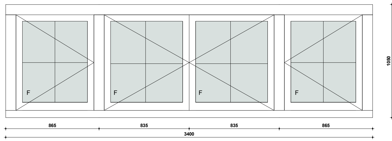
merk T - bestaand kozijn
