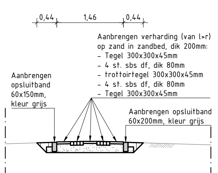
PRINCEPDETAIL 8 (Doorsteekjes Langestreek) Schaal 1:50
