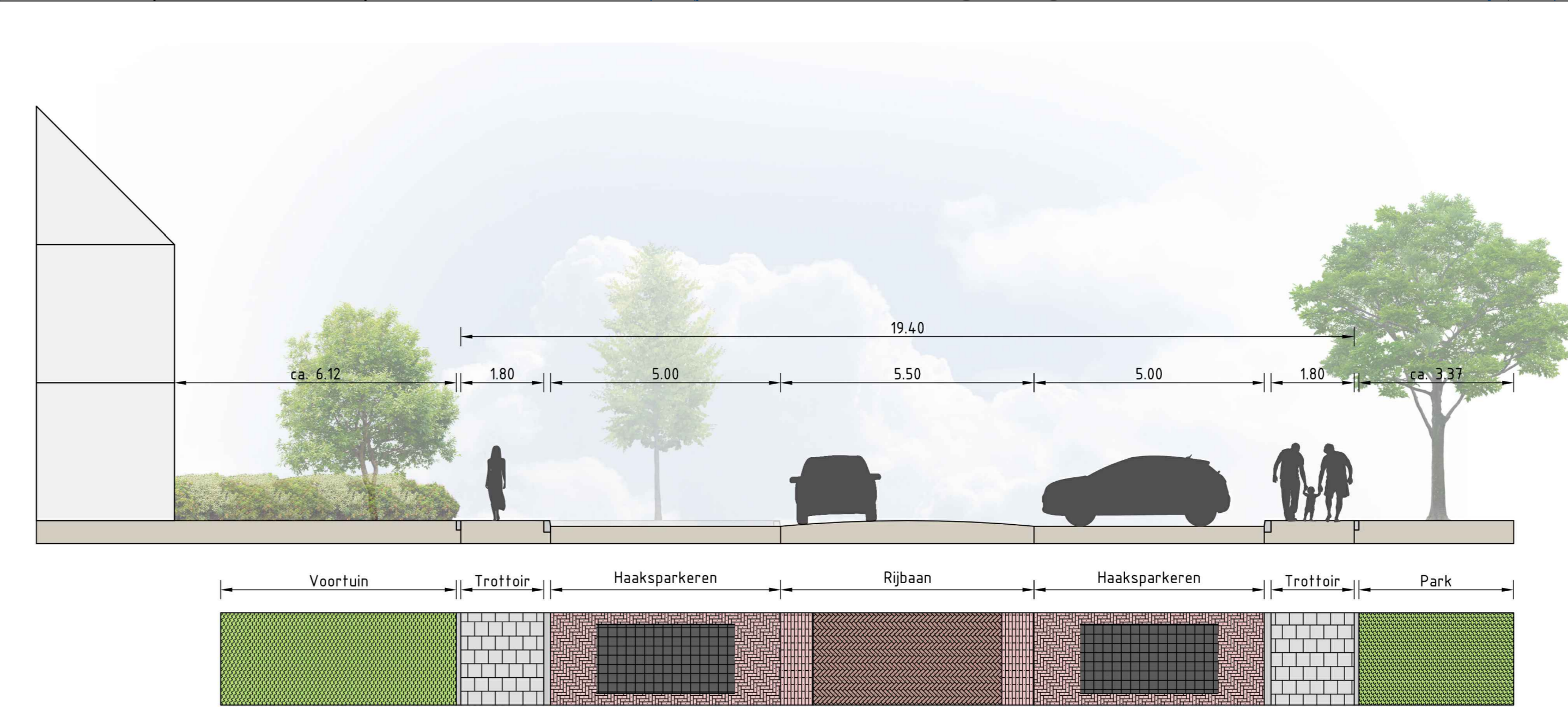
DWARSPROFIEL 03
