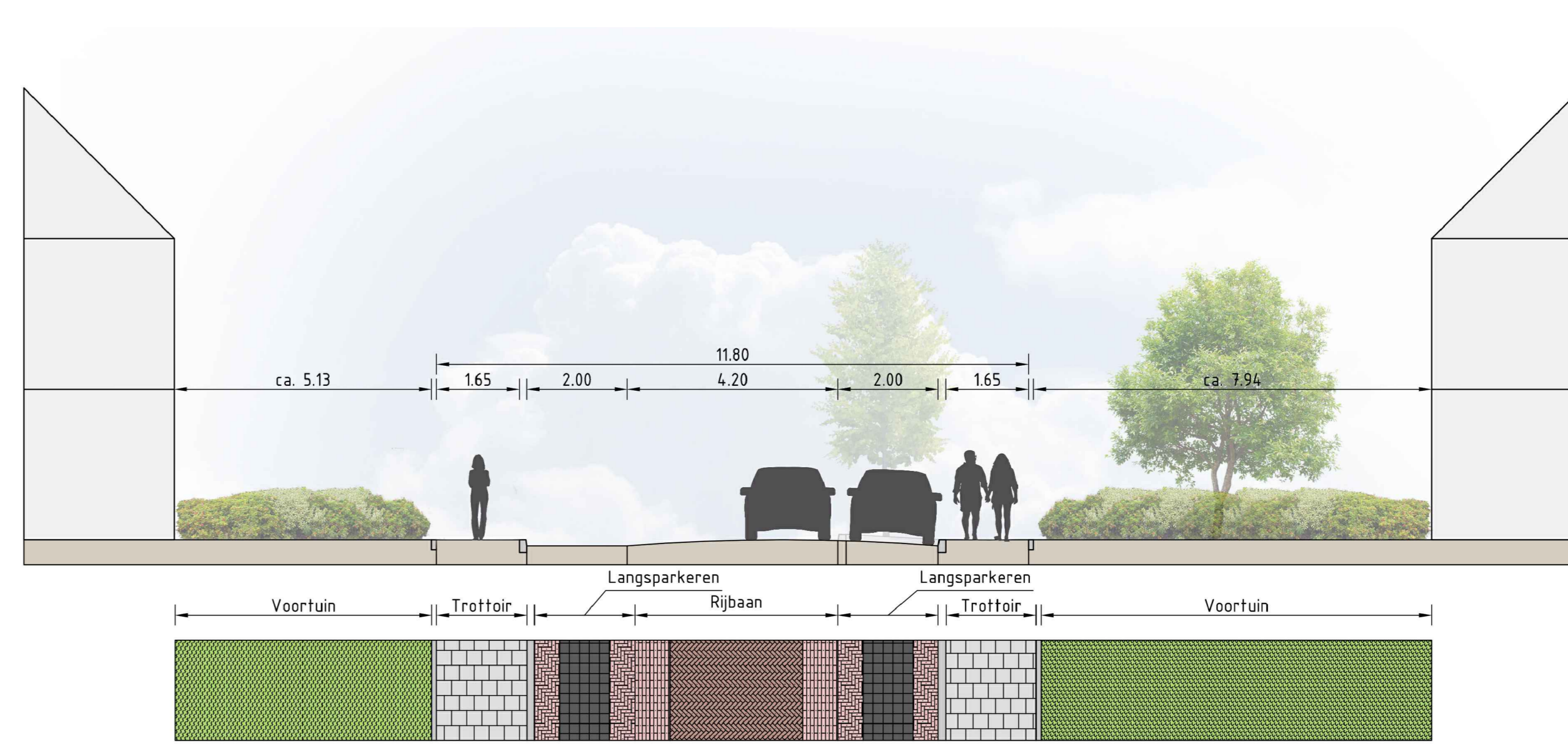
DWARSPROFIEL 02
