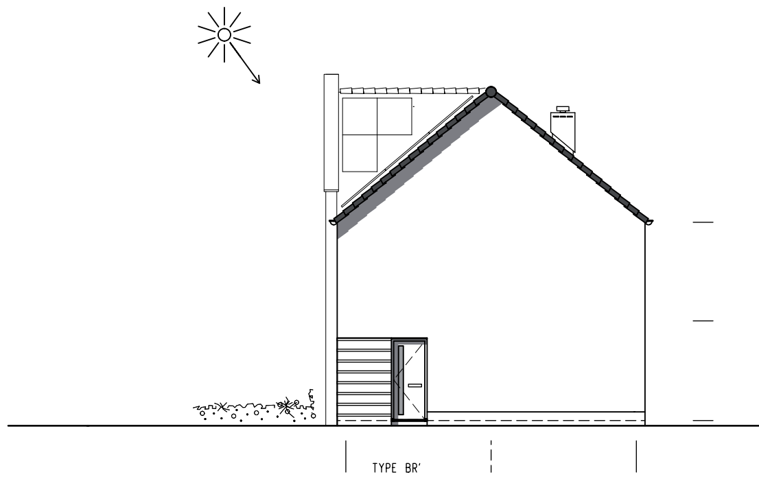
R. ZIJGEVEL Bouwnummer: 1.6
