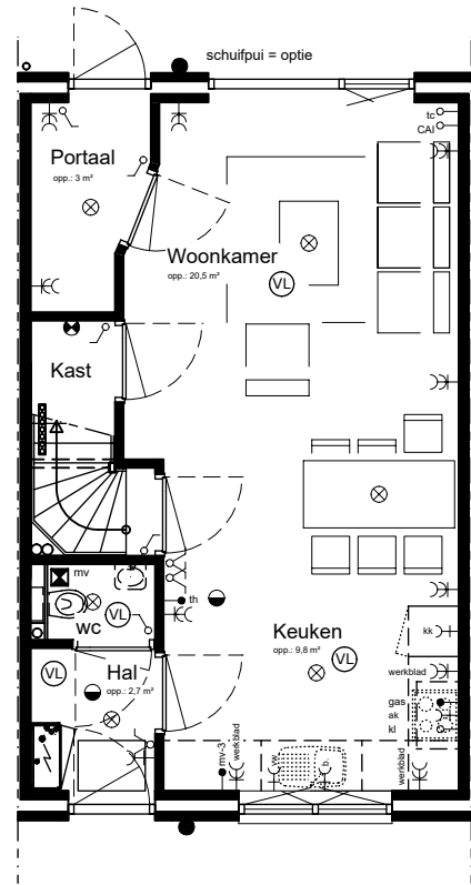
BEGANE GROND + OPTIE 3
