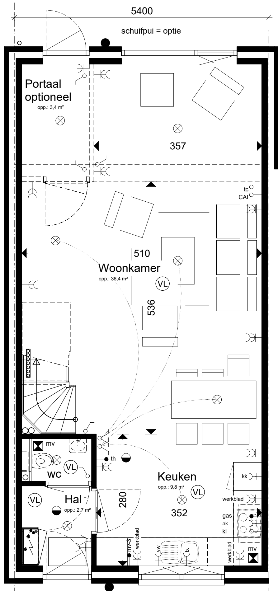
TYPE AL - UITBREIDING
