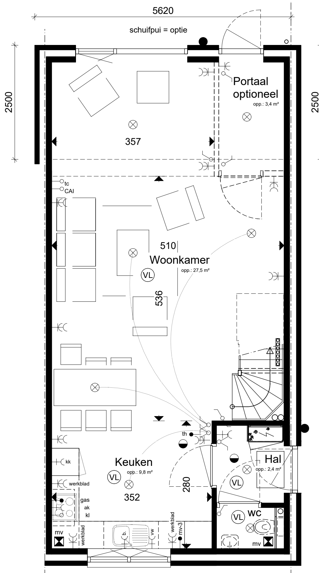
TYPE BR' - UITBREIDING
