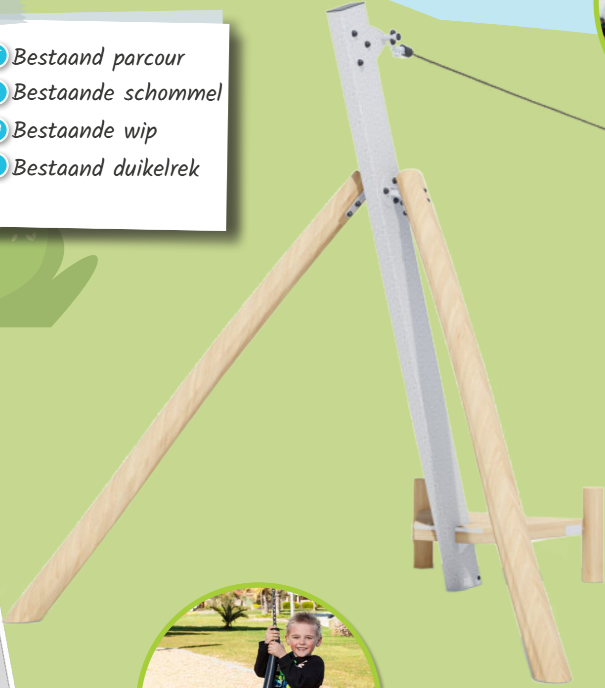
1 Kabelbaan
