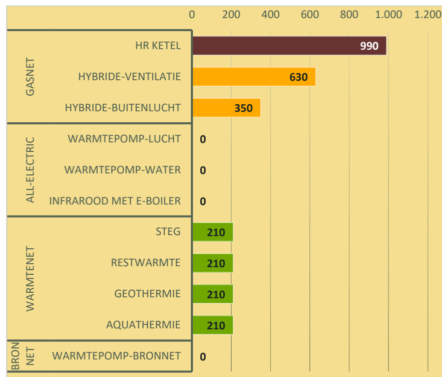
Figuur 2: Gasverbruik per techniek in m 3 /jaar, uitgesplitst naar techniek, voor een transitiegereede rijwoning 1950-1980. Gasverbruik in de elektriciteitsproductie en de hoofdbron van de STEG zijn in deze grafiek niet meegenomen.
