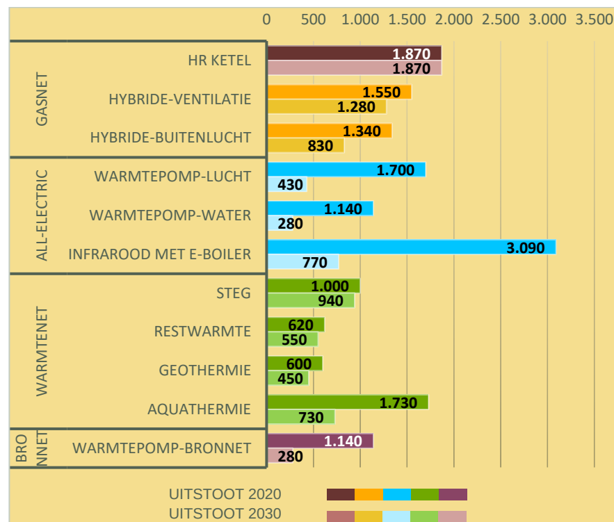
Figuur 3: CO 2 -uitstoot per techniek in kg, uitgesplitst naar techniek, in 2020 en 2030, voor een transitiegedere woning 1950-1980
