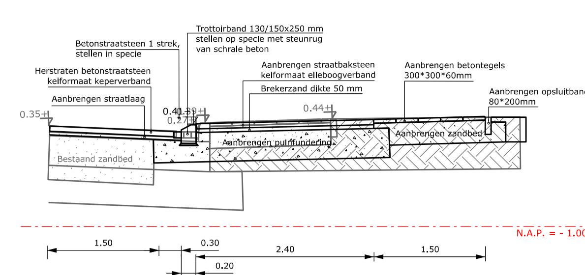
Dwarsprofiel B-B
