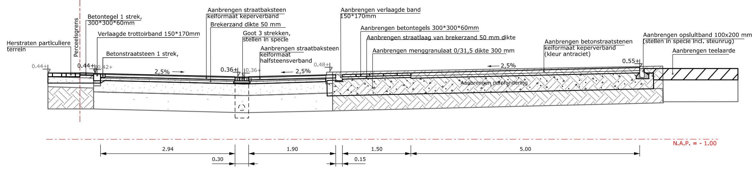
Dwarsprofiel A-A
