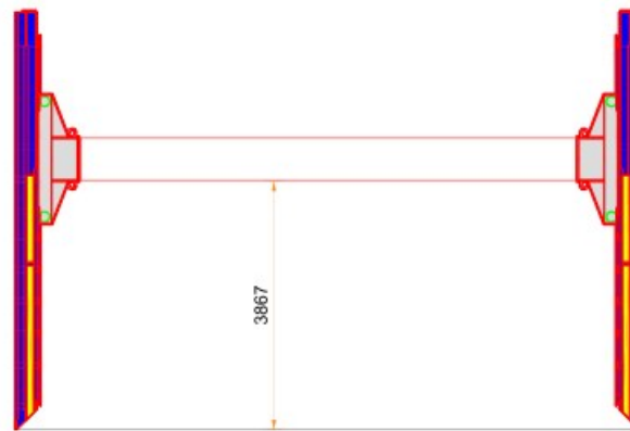
Doorsnede A-A
