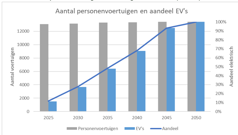
Figuur 8: Aandeel elektrische personenvoertuigen in Veere volgens EV Outlooks (ElaadNL)
