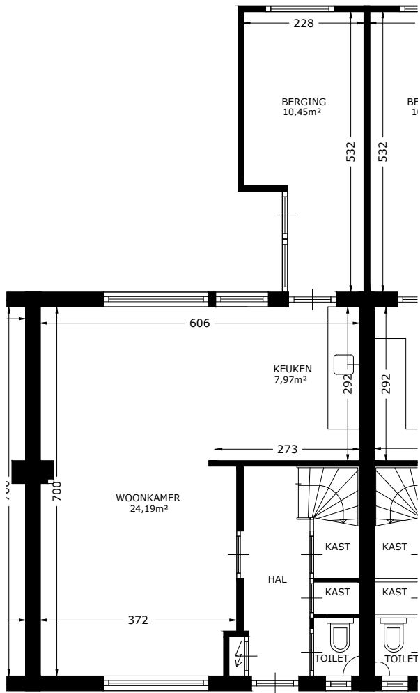
BEGANE GROND
