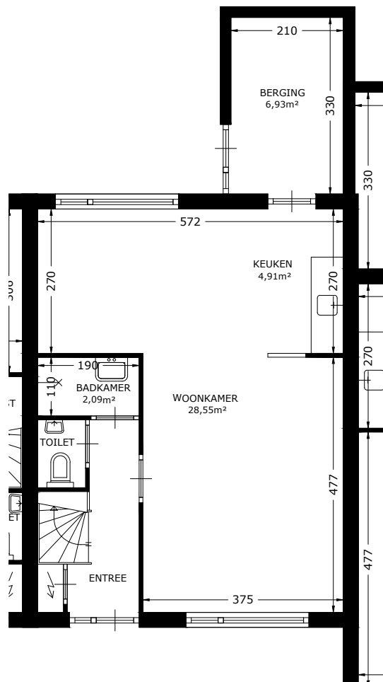
BEGANE GROND
