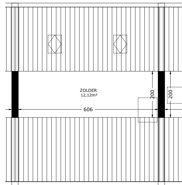
TWEEDE VERDIEPING
