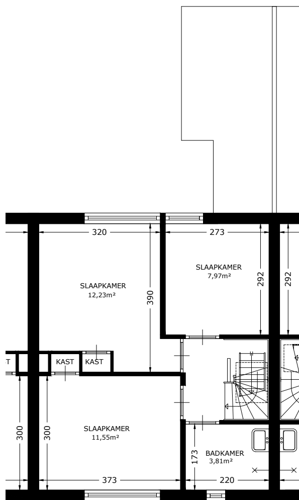
EERSTE VERDIEPING
