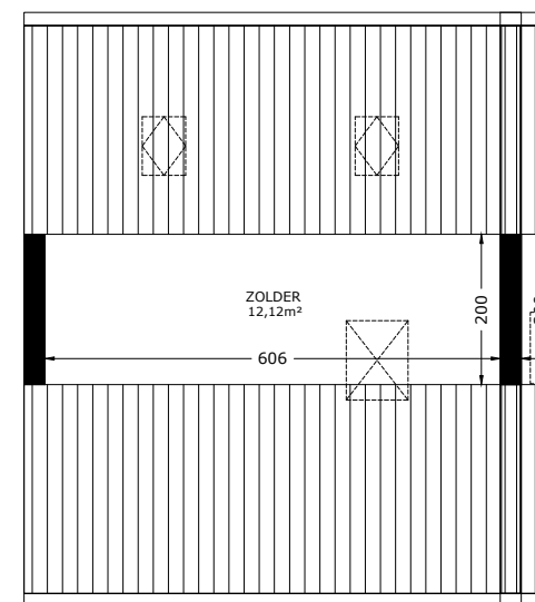
TWEDE VERDIEPING
