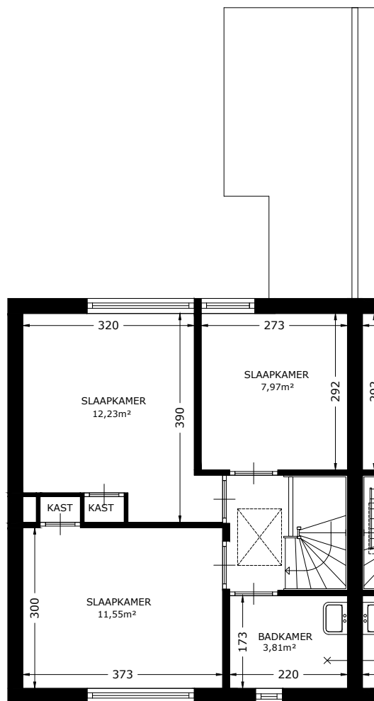
EERSTE VERDIEPING
