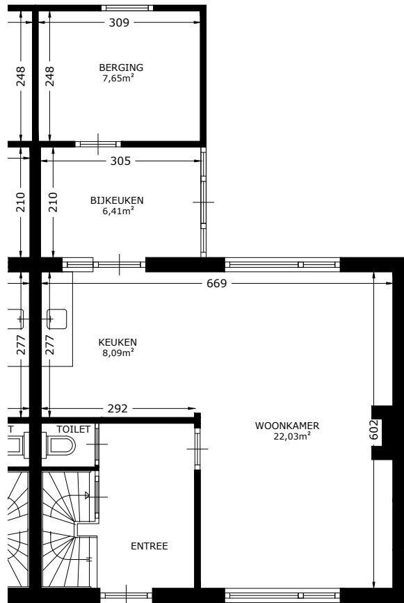
BEGANE GROND
