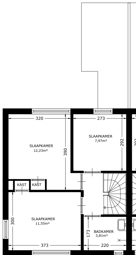
VERDIEPING
