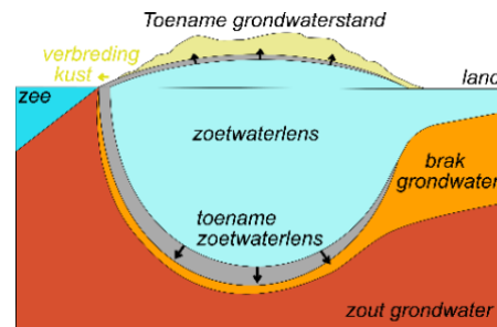
Figuur 14 Schematische weergave zoetwaterlens
