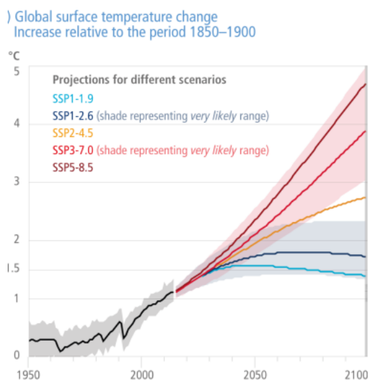
Figuur 1. Scenario's klimaatverandering (IPCC, 2022)
