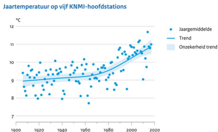
Figuur 4: Jaartemperatuur in Nederland van 1900-2020 (KNMI)
