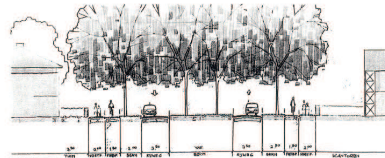
Dwarsprofiel hoofdontsluiting
