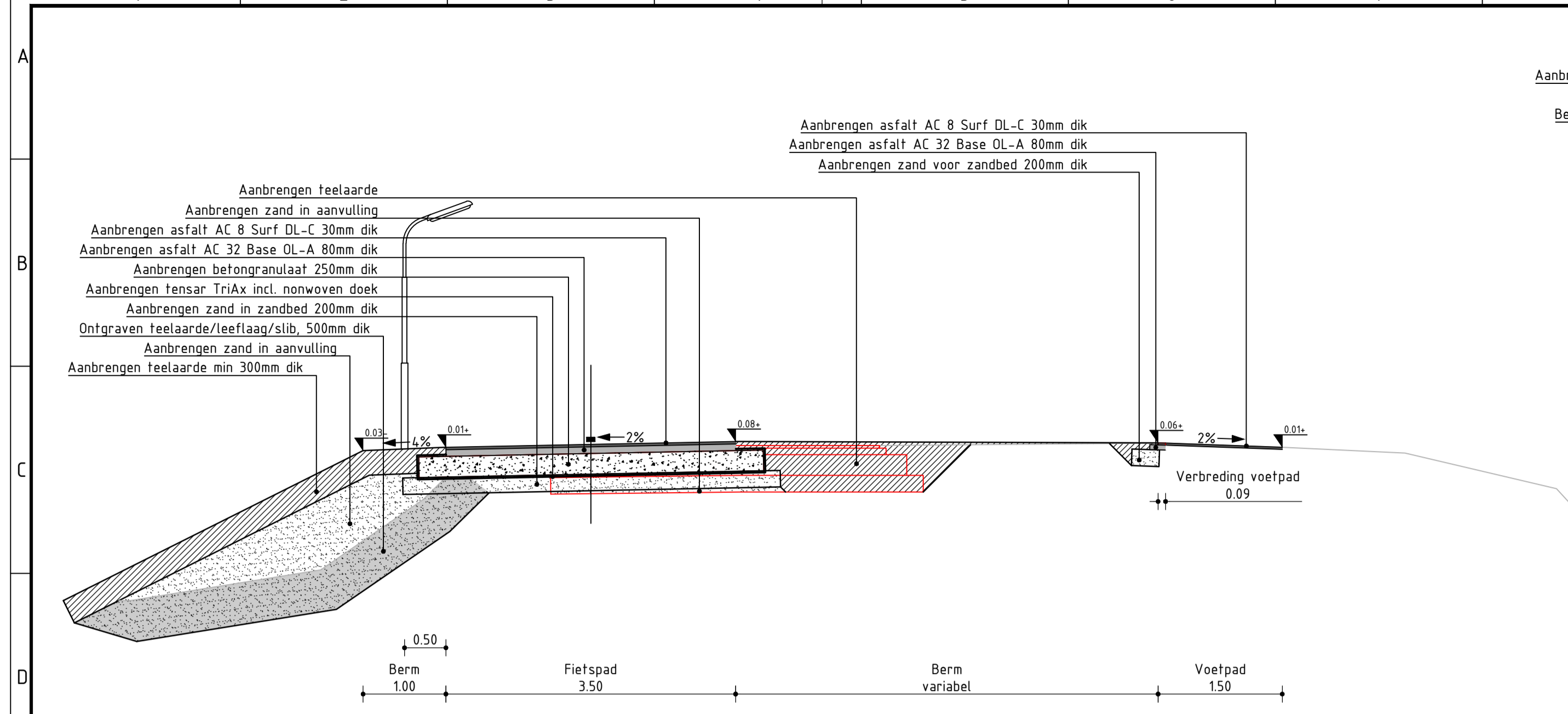
Normaalprofiel D1-D1 Schaal 1:50
