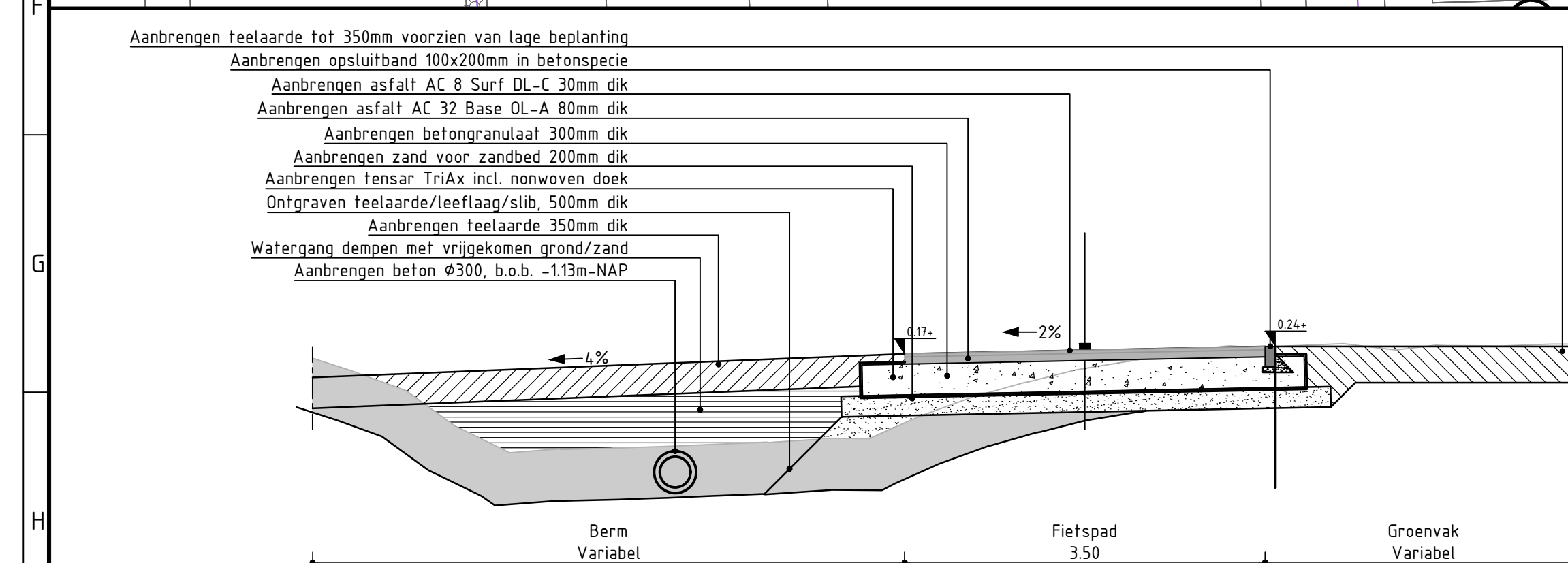
Normaalprofiel F-F Schaal 1:50
