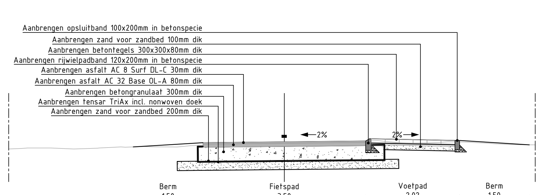
Normaalprofiel G-G Schaal 1:50
