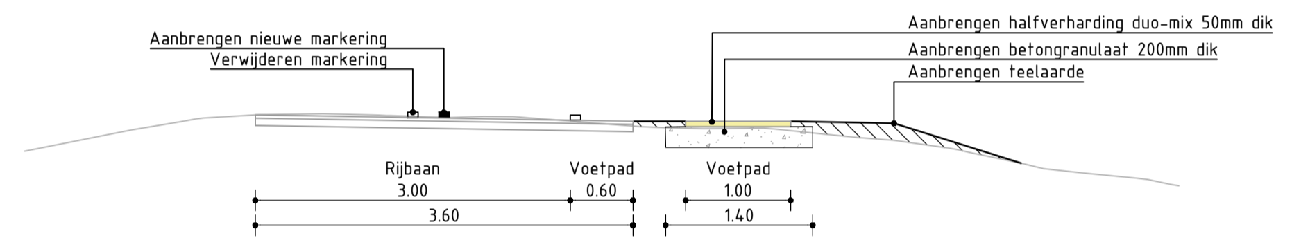
Normaalprofiel K1-K1 Schaal 1:50
