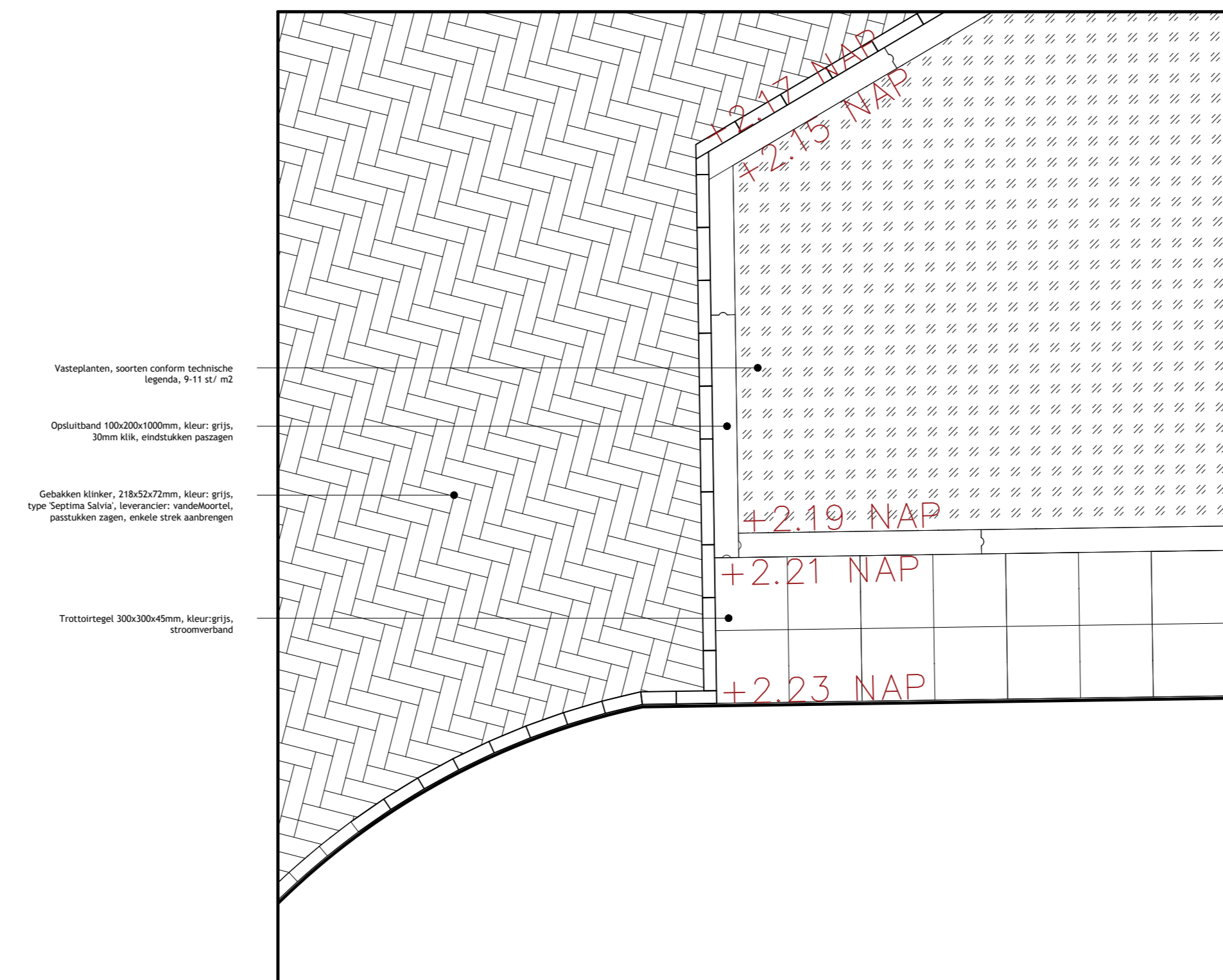
Detail 1.2 (schaal 1:20)
