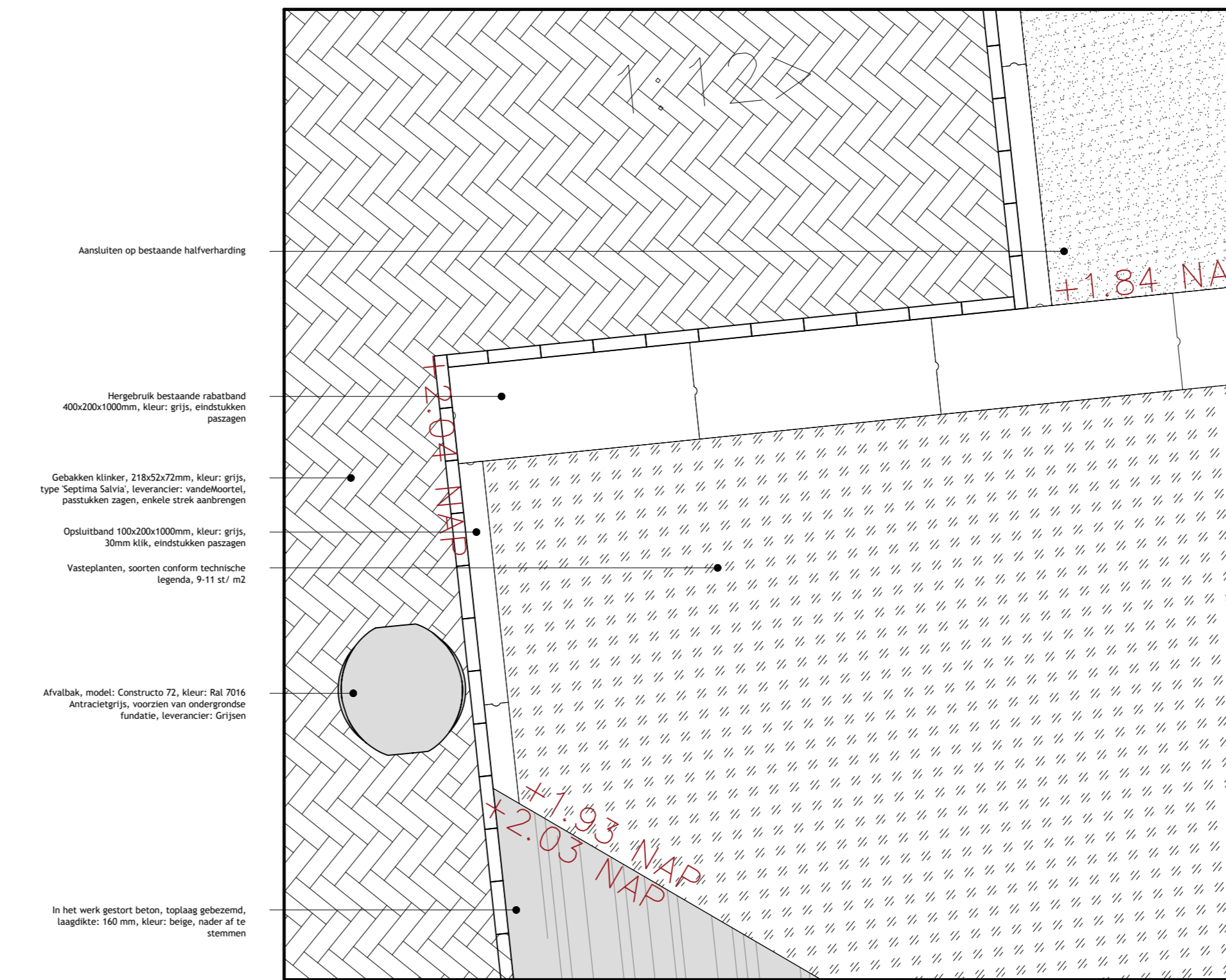
Detail 1.3 (schaal 1:20)
