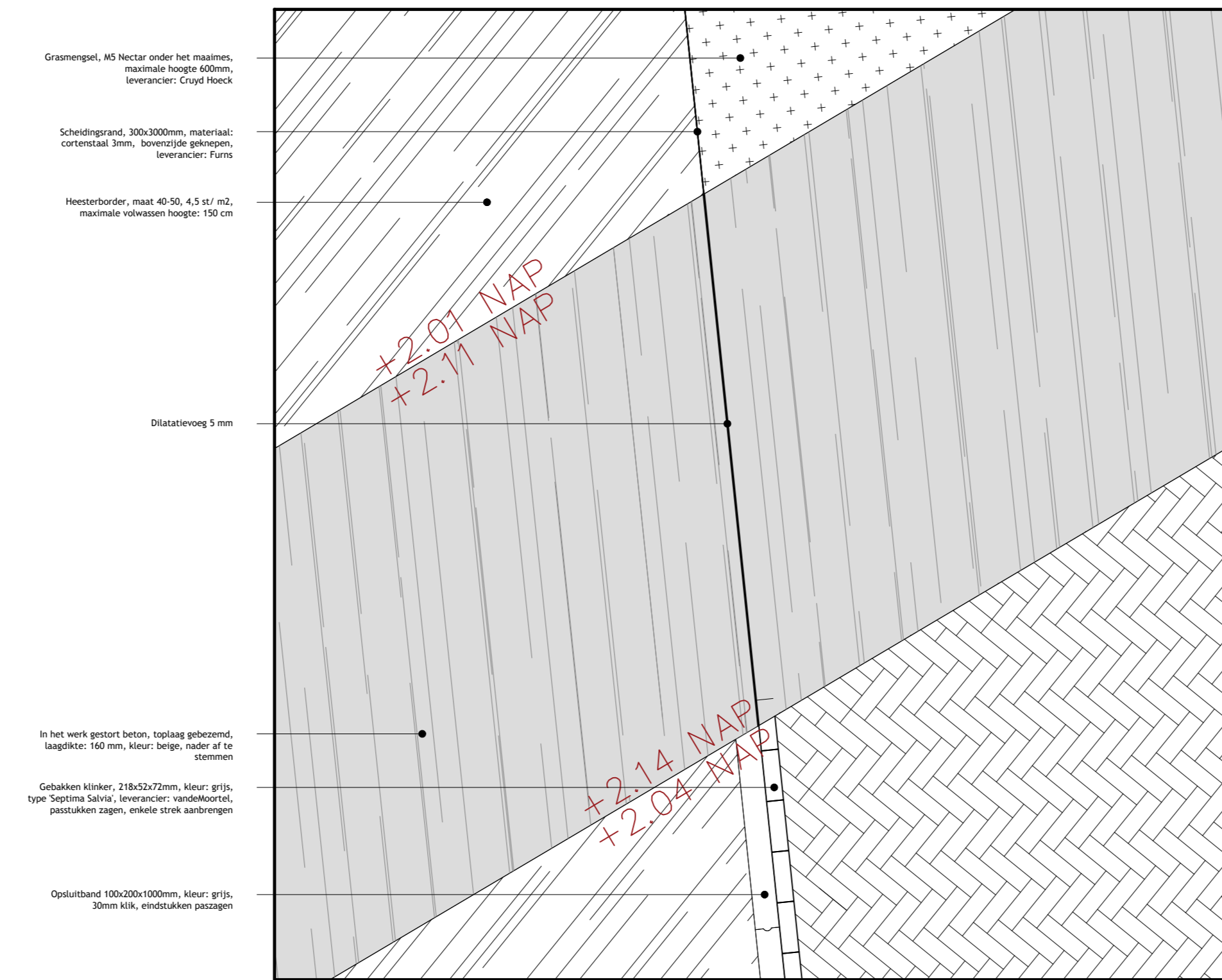
Detail 1.1 (schaal 1:20)
