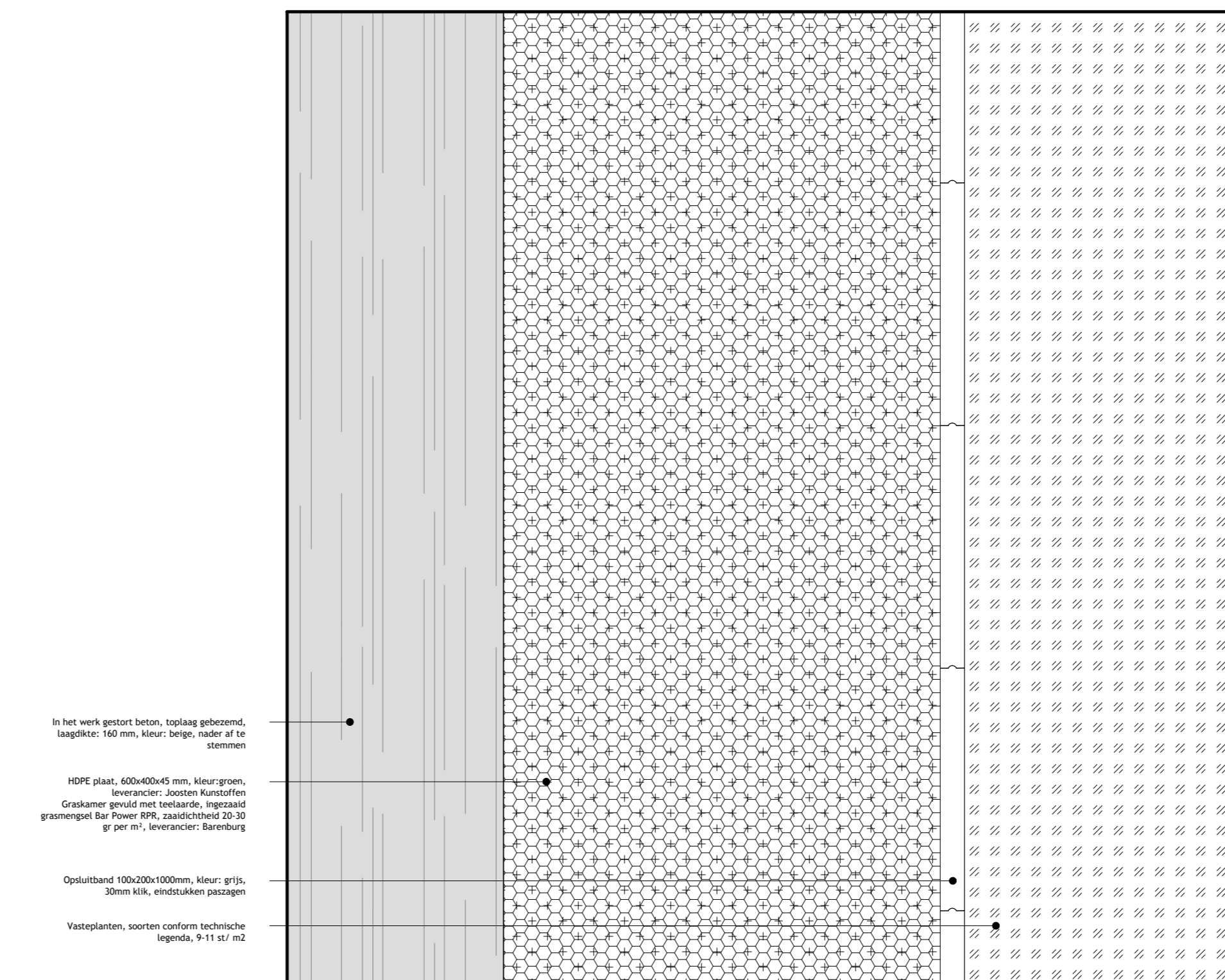
Detail 1.4 (schaal 1:20)
