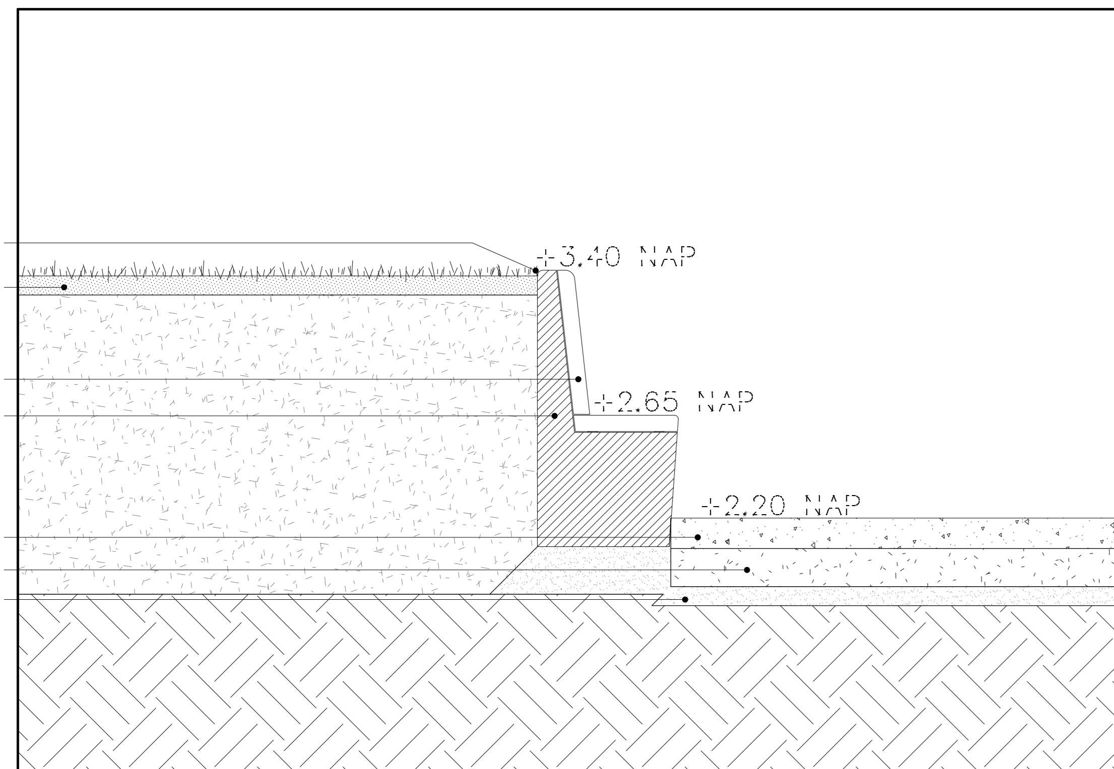
Principeprofiel 1.2 Grondkerend meubel (schaal 1:20)
