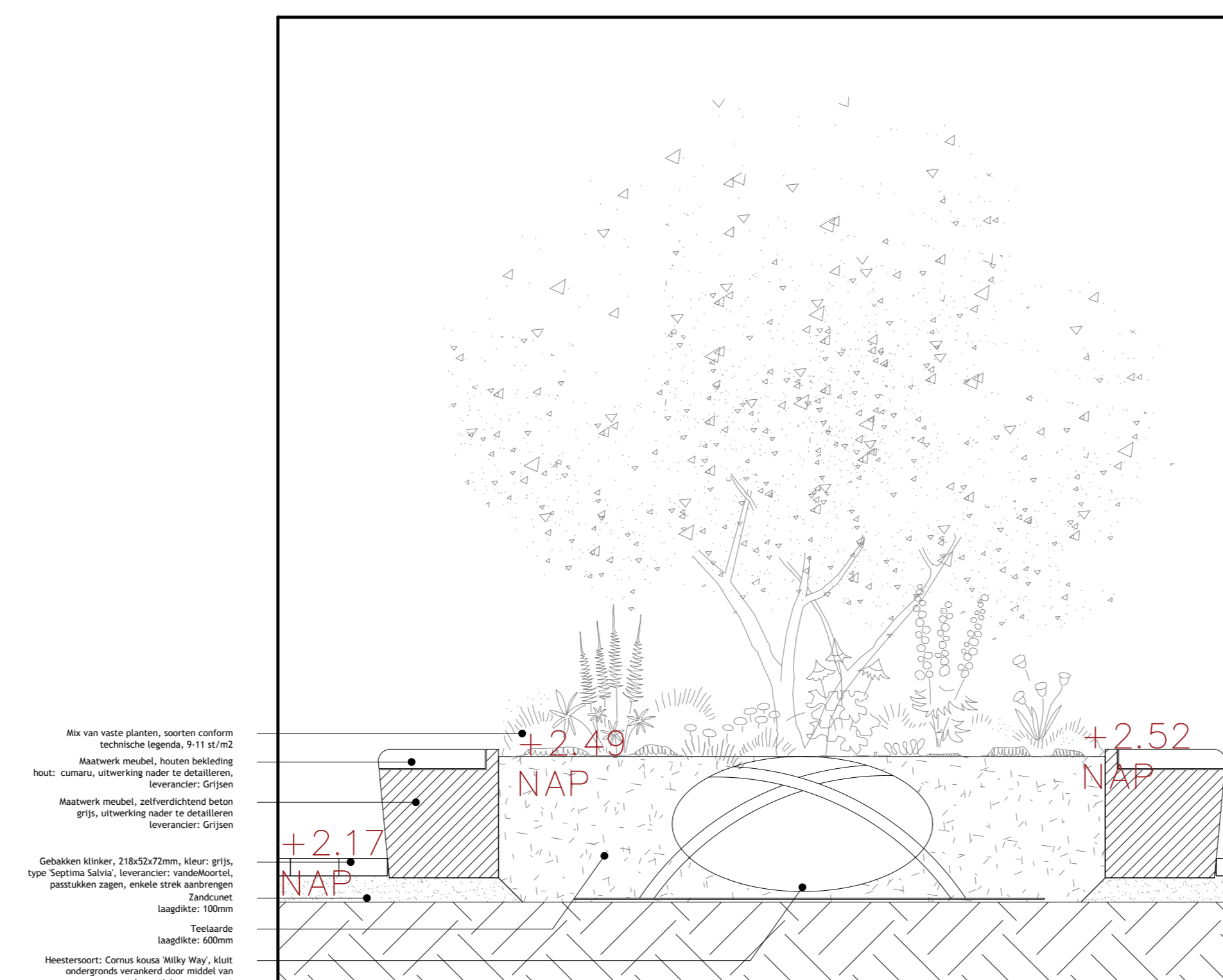
Principeprofiel 1.4 Meubel Leest (schaal 1:20)
