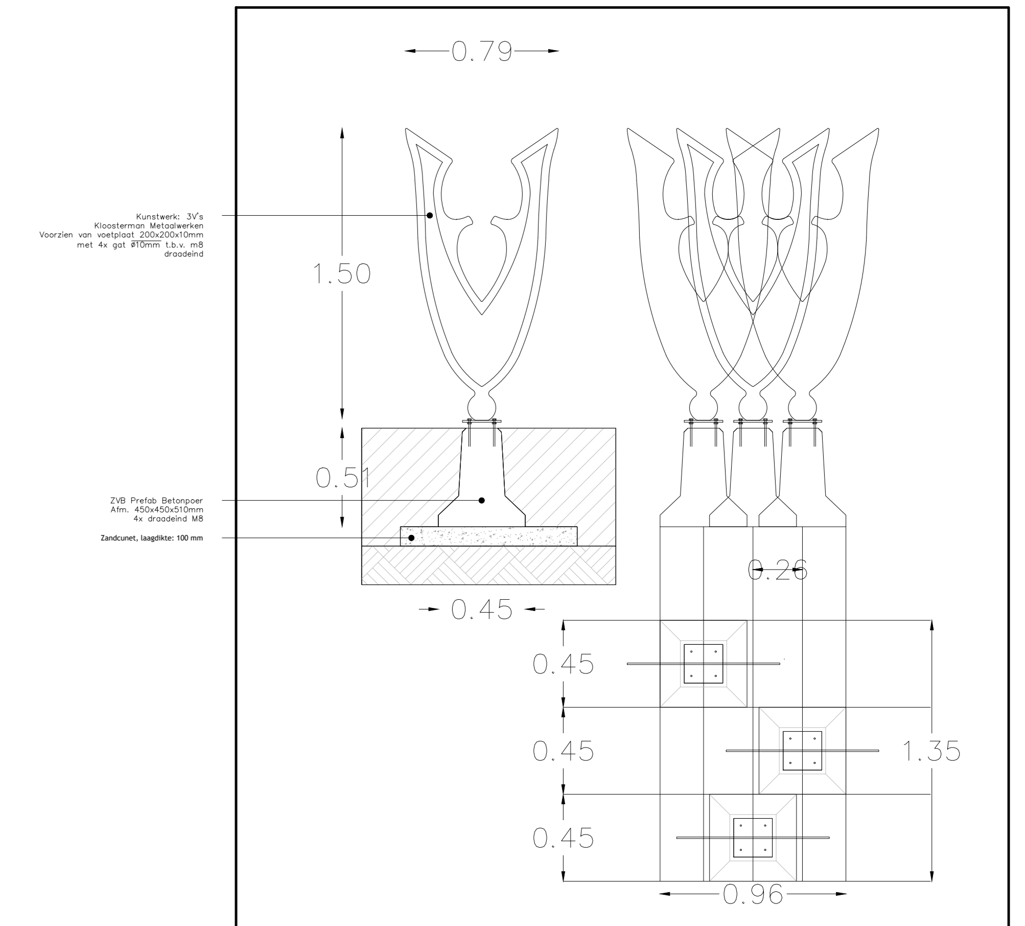
Detail 1.5 (schaal 1:20)
