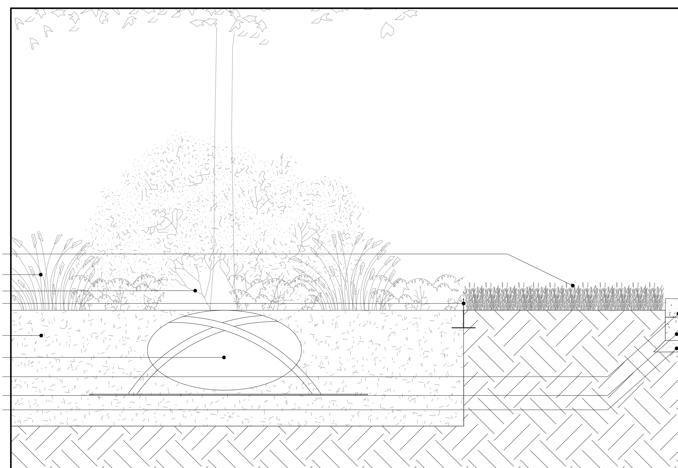
Principeprofiel 1.3 Slagenlandschap (schaal 1:20)
