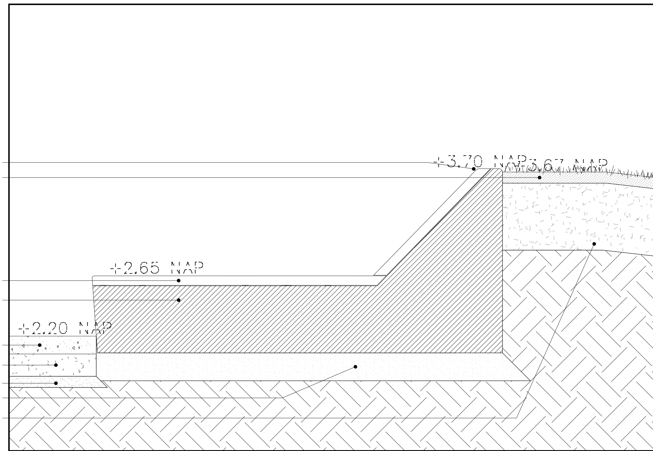
Principeprofiel 1.1 Zitmeubel (schaal 1:20)
