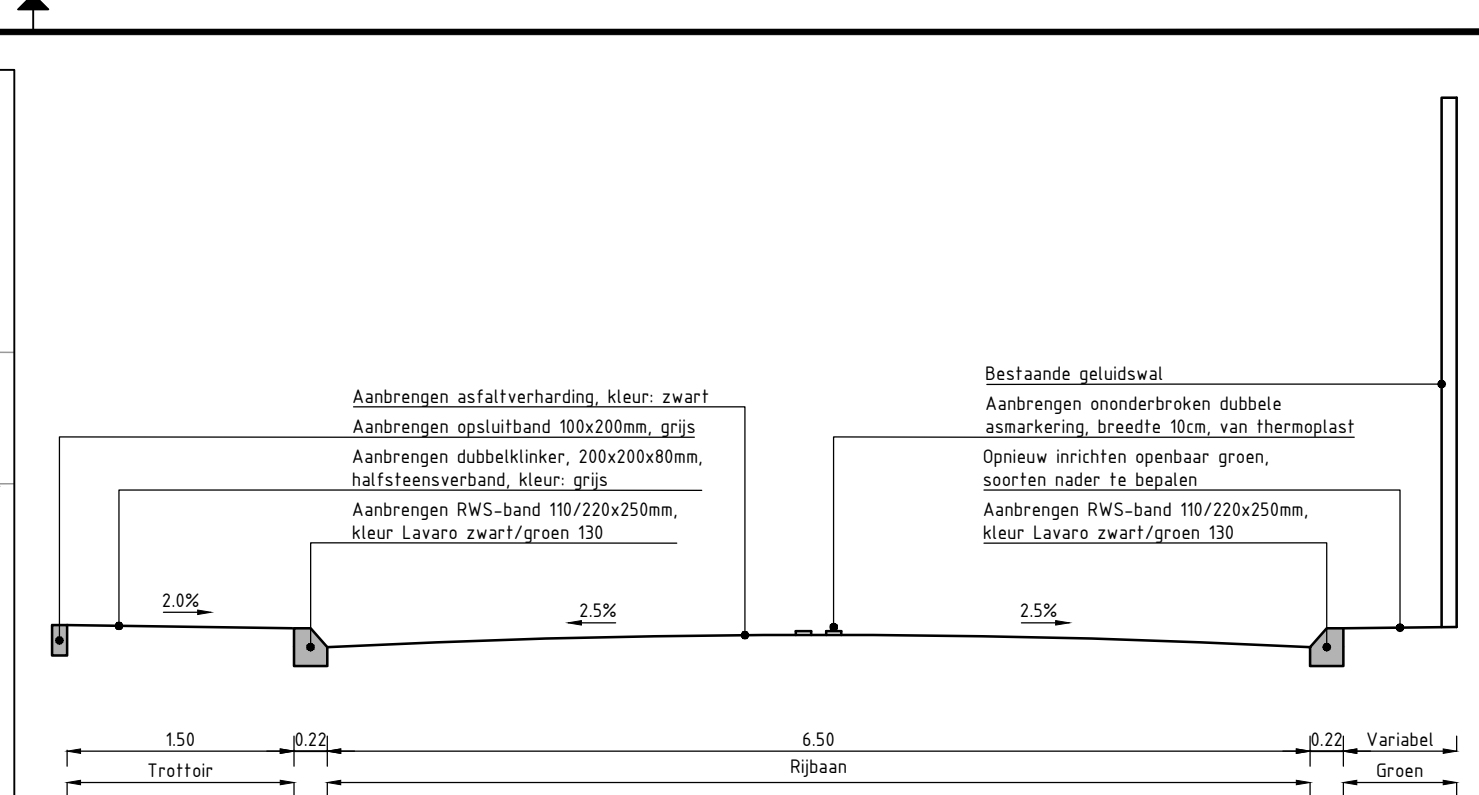
Principe profiel 1 Schaal 1:50
