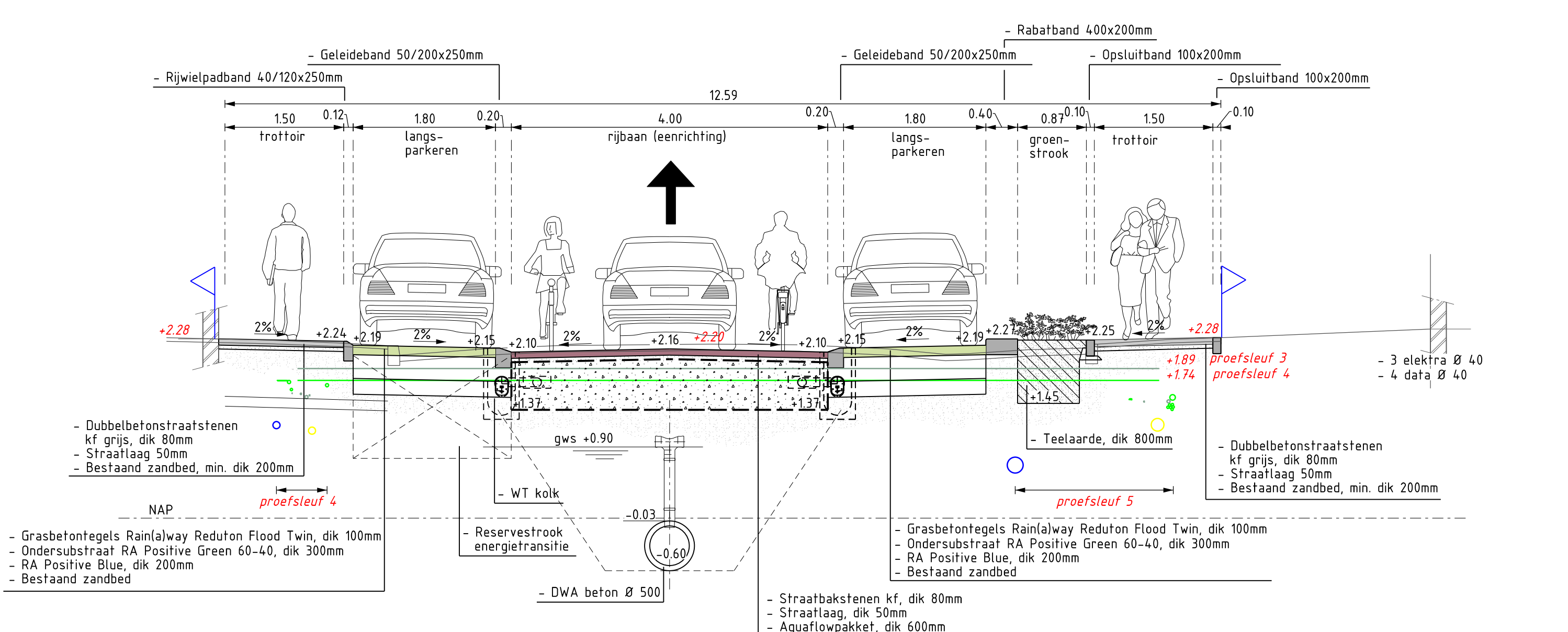
DWARSPROFIEL 1 schaal 1:50
