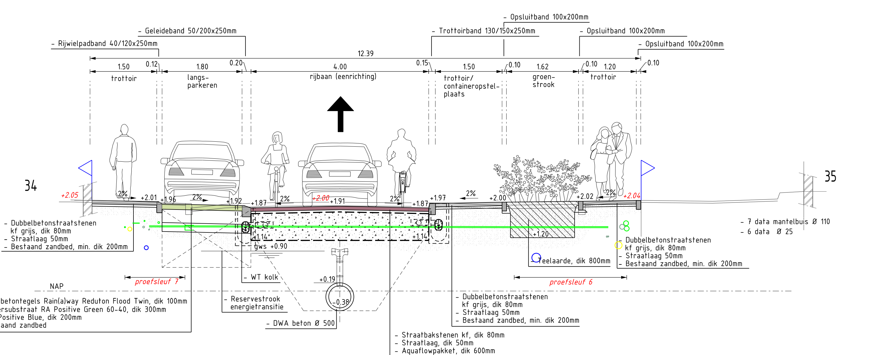
DWARSPROFIEL 2 schaal 1:50
