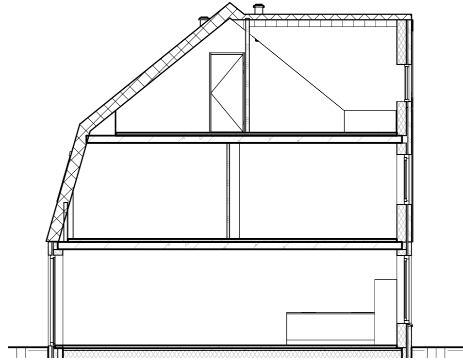
doorsnede B, 1:100
