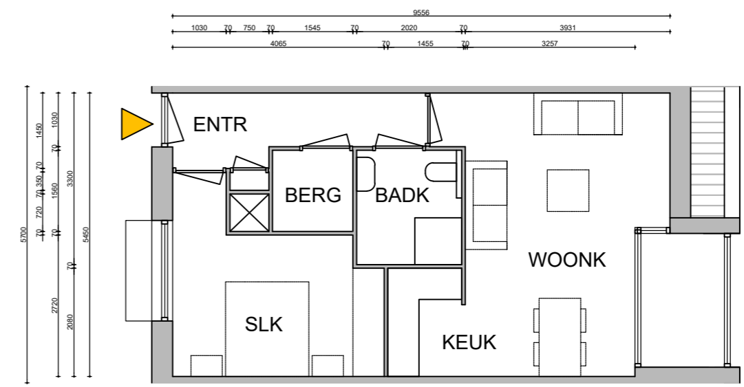
BASIS TWEEKAMER STARTERSWONING ONDER KAP
