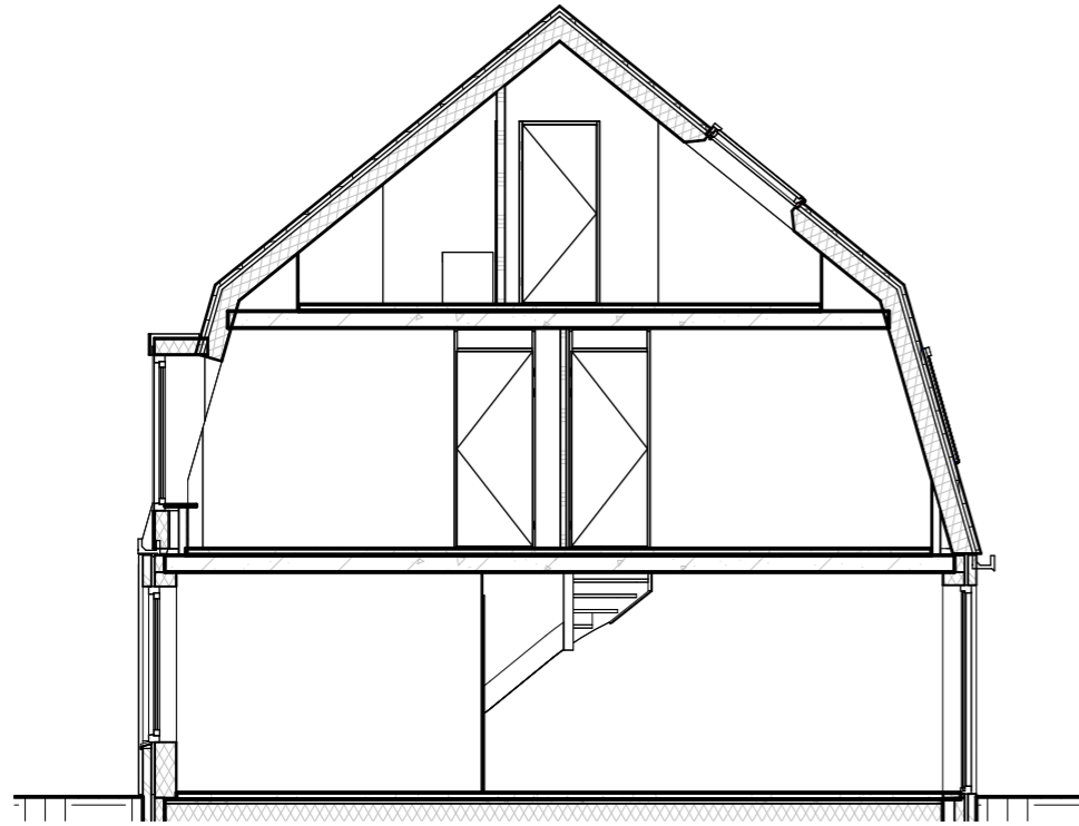
doorsnede A, 1:100
