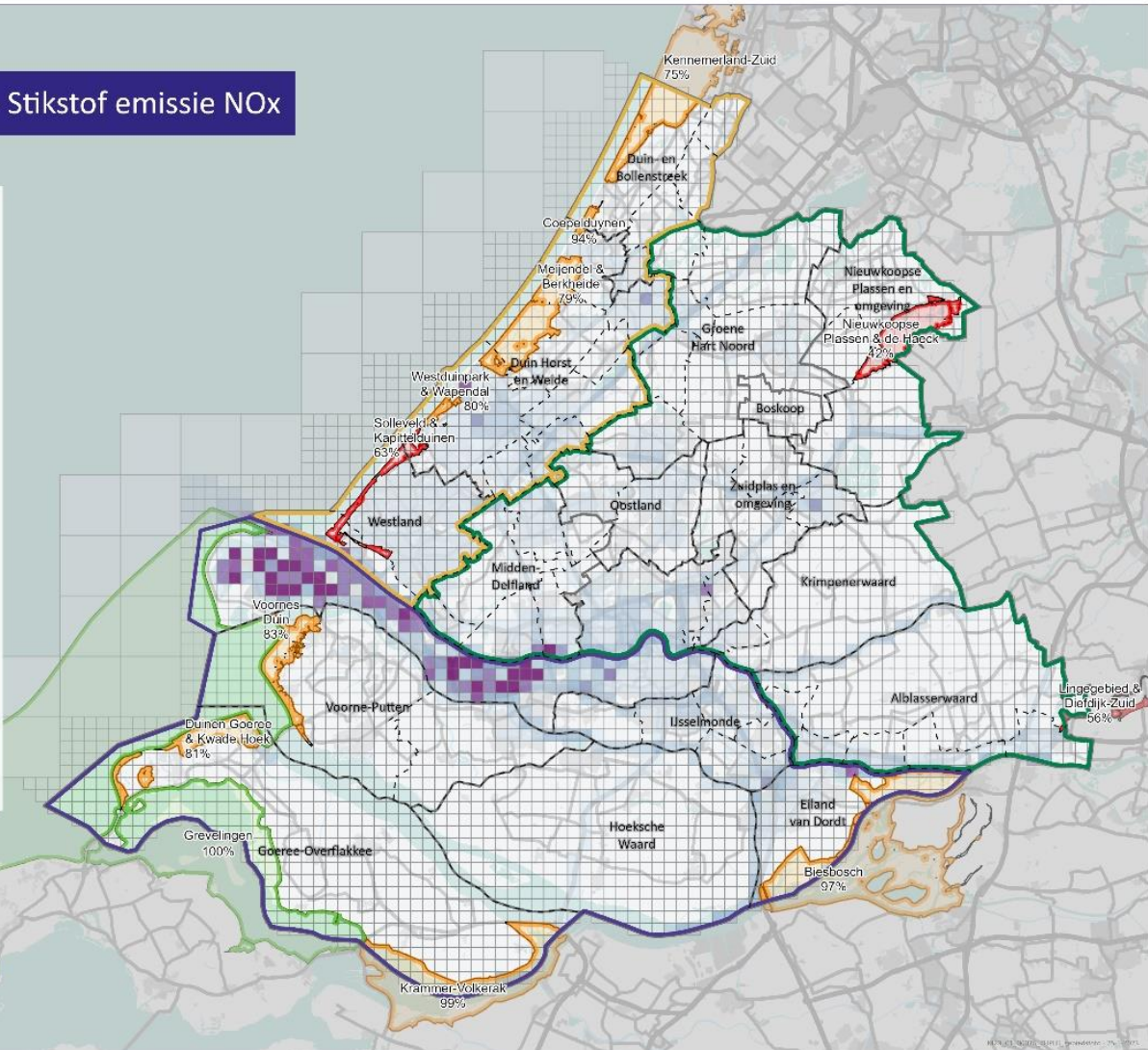
Kaart 10: emissie NOx en stikstofgevoelige natuur
