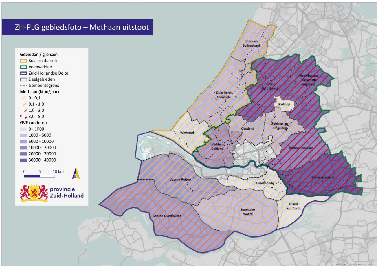
Kaart 13: emissie van methaan door veeveelt in Zuid-Holland
