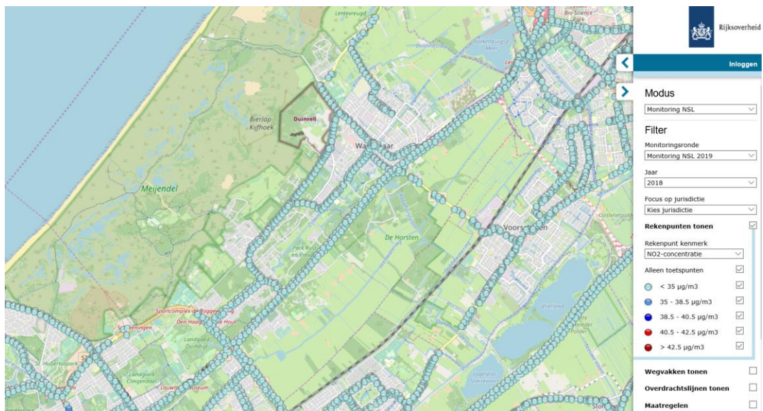
Figuur 3.2 Jaargemiddelde concentratie NO 2 in 2018 (NSL monitoringstool)
