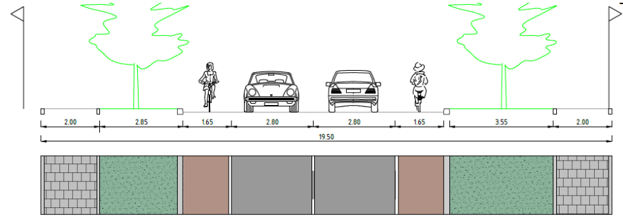
Principeprofiel 26 Van der Oudermeulenlaan: Bestaande situatie Schaal: 1:100
