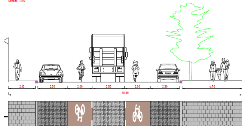
Principeprofiel 06 Johan de Wittstraat: Nieuwe situatie
