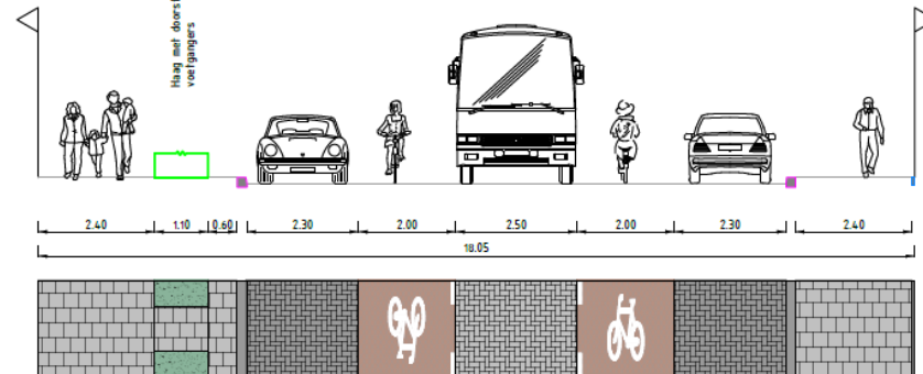
Principeprofiel 12 Bellesteynlaan: Nieuwe situatie Schaal: 1:100
