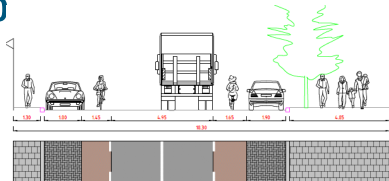
Principeprofiel 06 Johan de Wittstraat: Bestaande situatie
