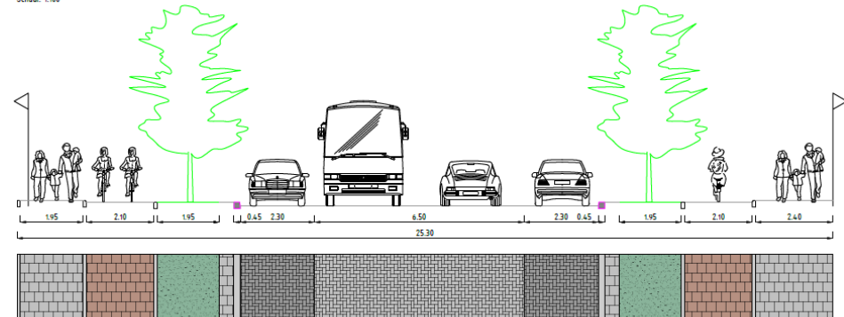
Principeprofiel 16A Storm van 's-Gravensandeweg. Nieuwe situatie Schaal: 1:100
