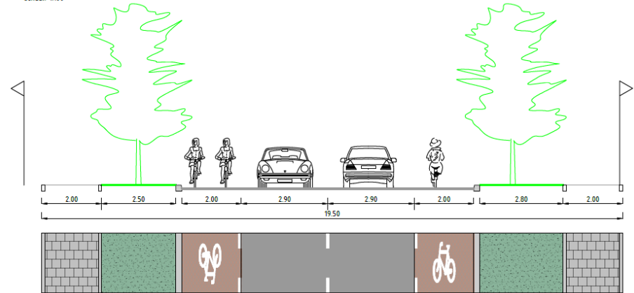
Principeprofiel 26 Van der Oudermeulenlaan: Nieuwe situatie (GOW50) Schaal: 1:100
