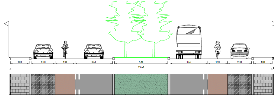
Principeprofiel 21 Prinsenweg: Besteande situatie Schaal: 1:100
