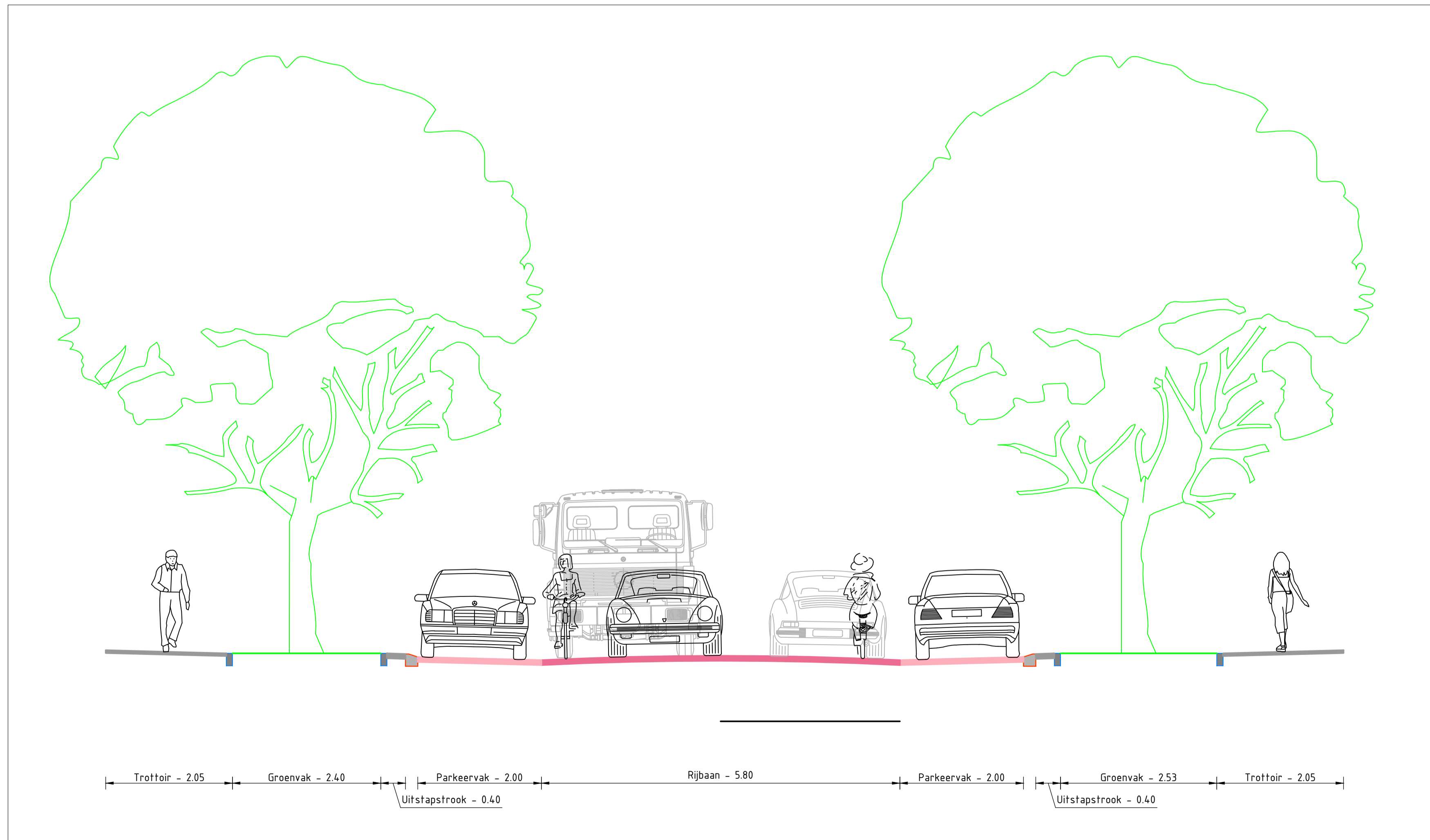
Nieuwe dwarsdoorsnede Schaal 1:50
