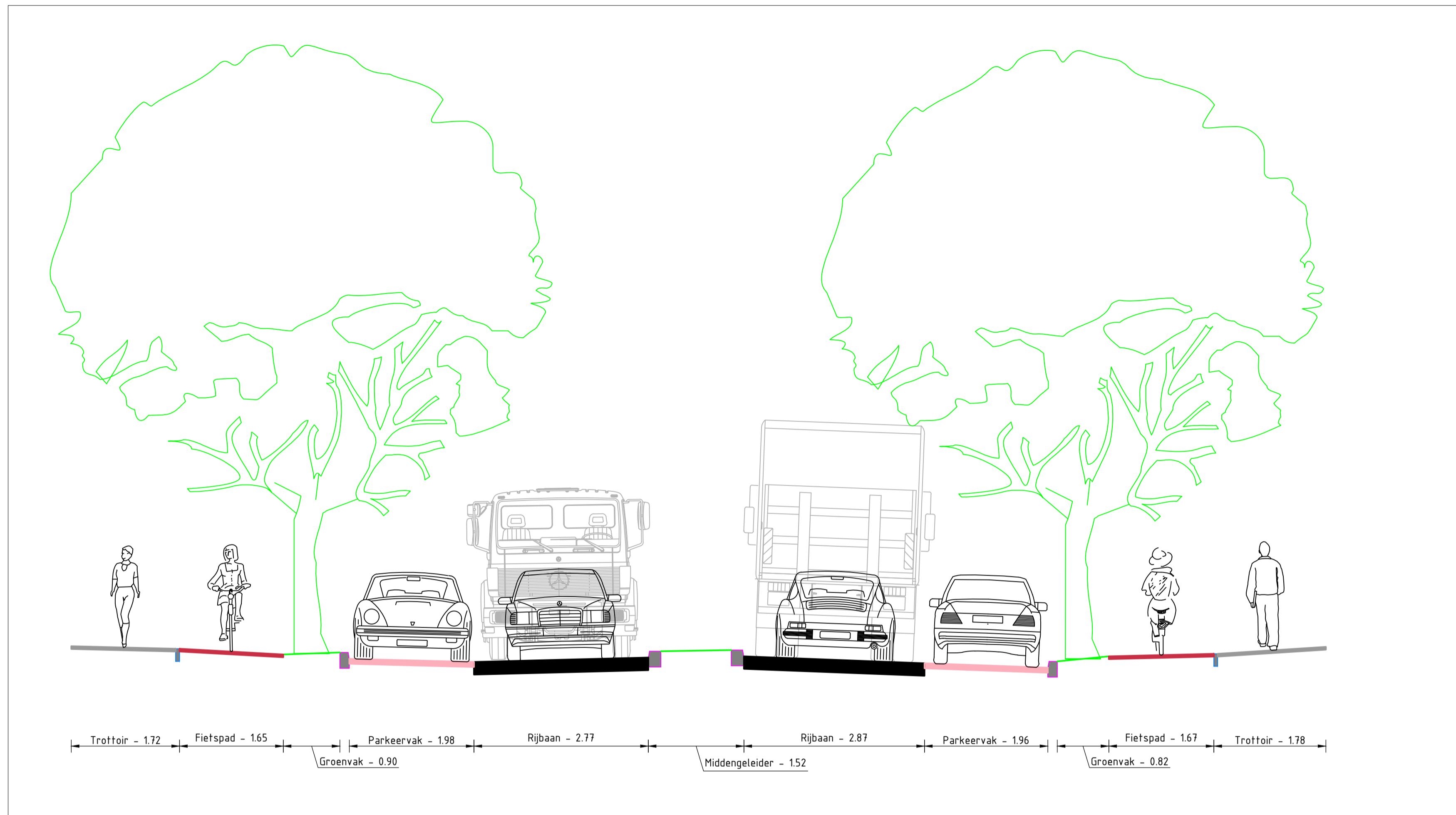
Bestaande dwarsdoorsnede Schaal 1:50
