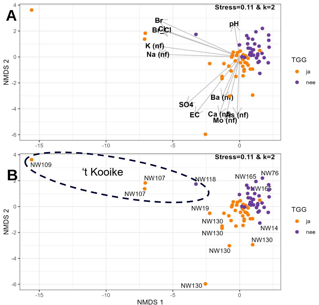
Figuur 4.15. NMDS plot voor meetpunten in Noordwaard gebaseerd op de TGG indicatorstoffen: "EC", "pH", "Br", "Br:Cl verhouding", "Cl", "SO 4 ", "Ca (nf)", "K (nf)", "Na (nf)", "As (nf)", "Mo (nf)", "Ba (nf)". Elk punt representeert een meting op een bepaalde meetlocatie. De pijlen geven de associatie met een bepaalde stof aan, hoe langer de pijl hoe sterker de associatie (hogere concentraties). Onderliggende concentraties zijn geschaald. In Figuur B is dezelfde NDMS plot weergegeven maar dan is bij de extremere punten aangegeven om welke meetlocaties het gaat.
