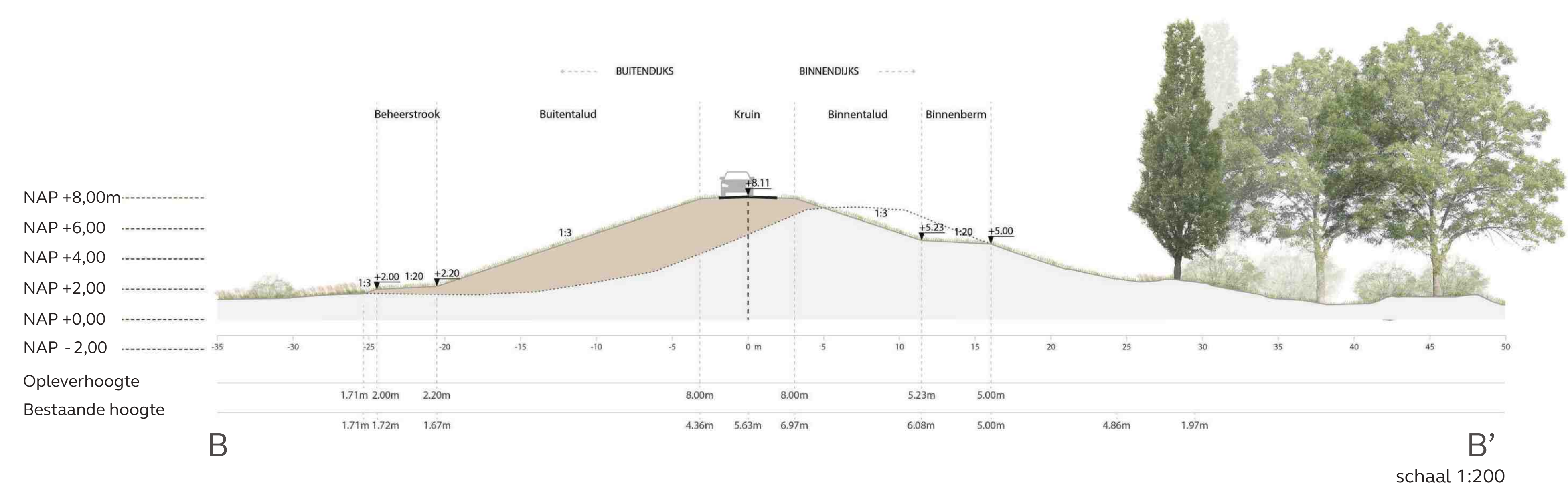
Profiel BB' Kruinverhoging en buitenwaartse asverschuiving
