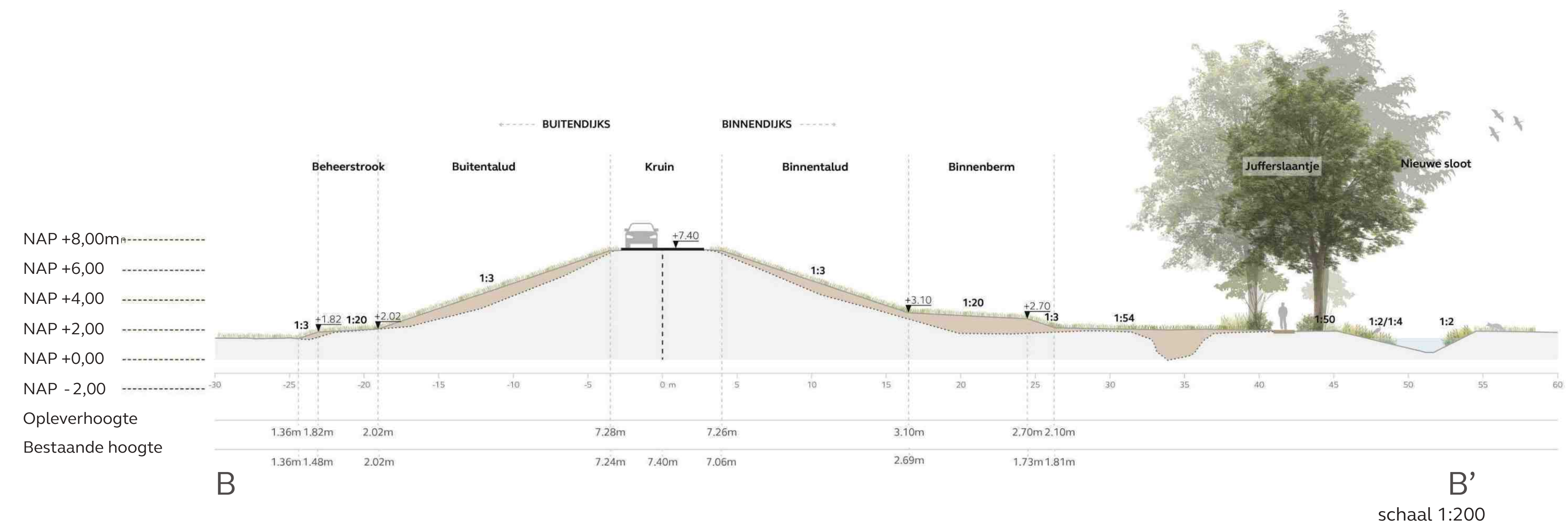
Profiel BB' Binnenwaartse berm en Jufferstaantje naast berm
