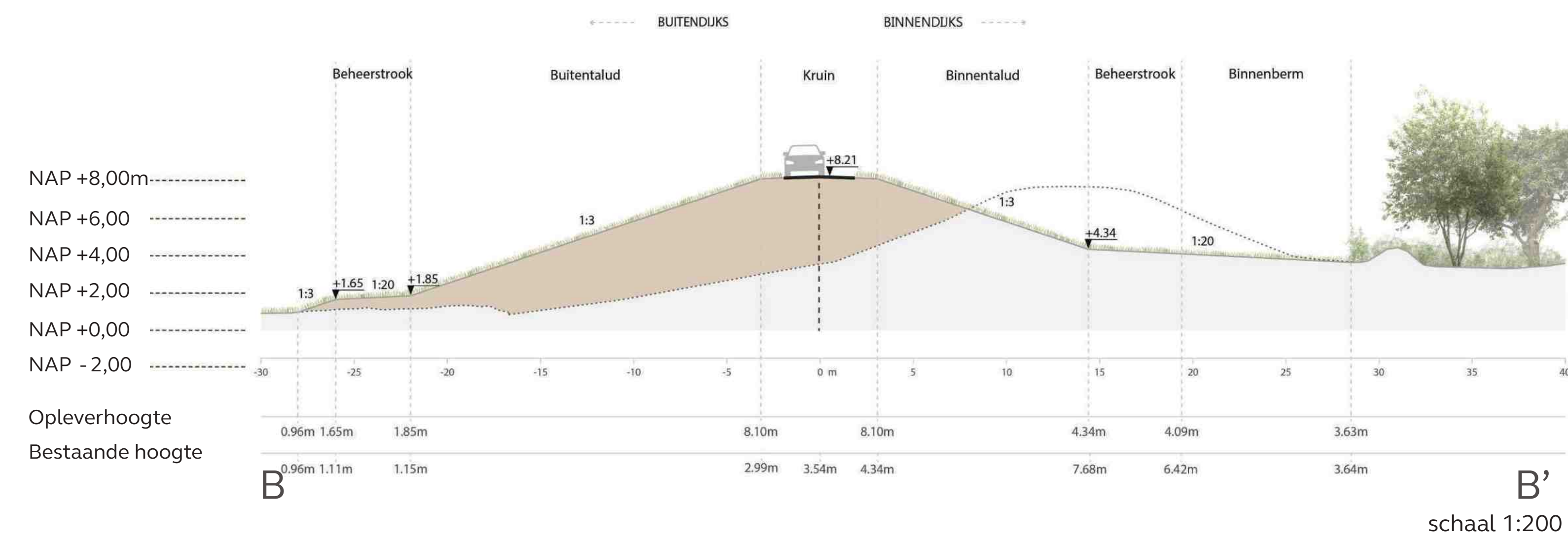
Profiel CC' Kruinverhoging en buitenwaartse asverschuiving
