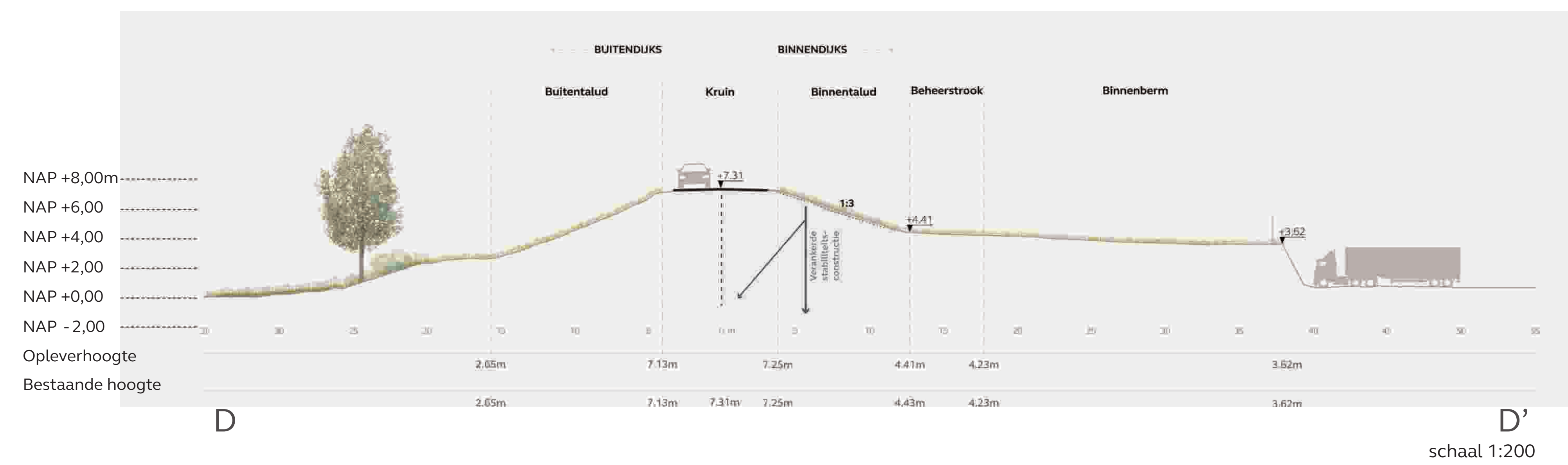
Profiel DD' Constructie stabiliteit
