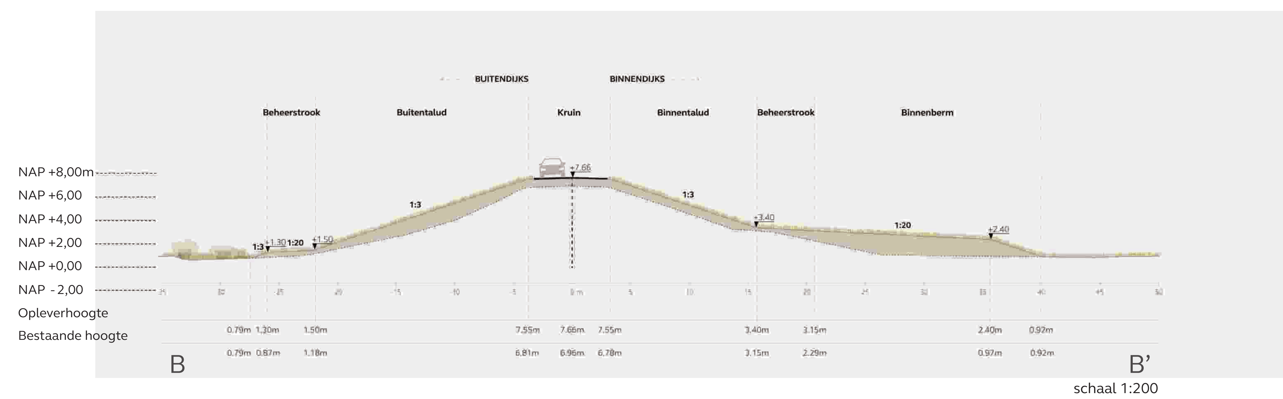
Profiel BB' Kruinverhoging en binnenberm
