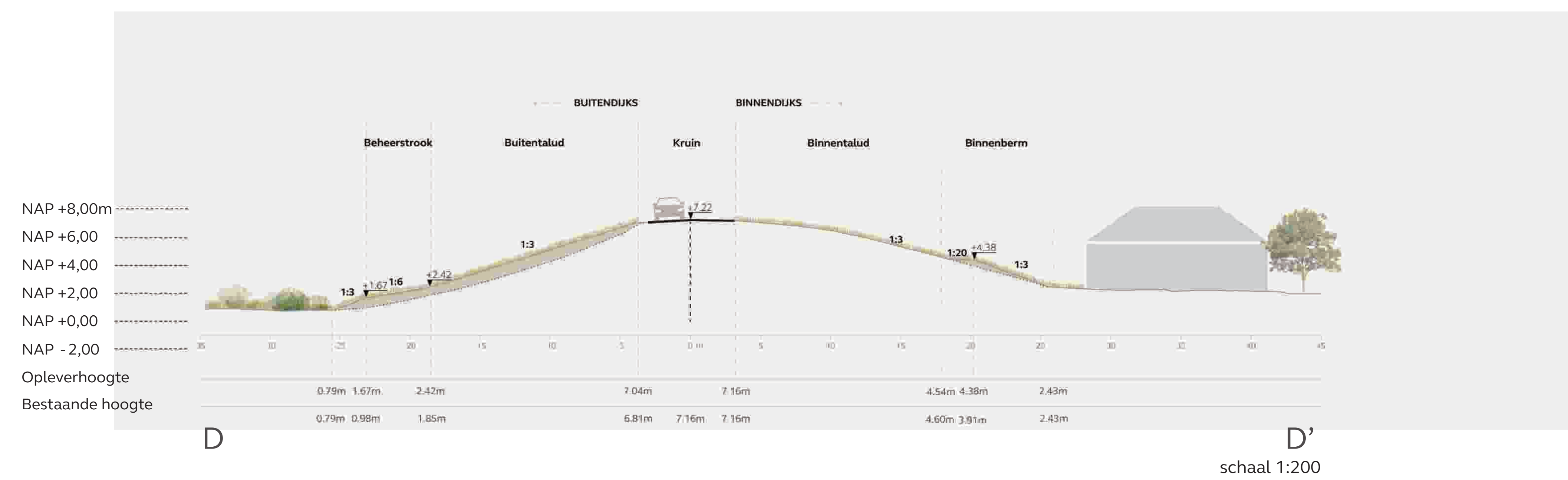
Profiel DD' Verflauwing buitentalud
