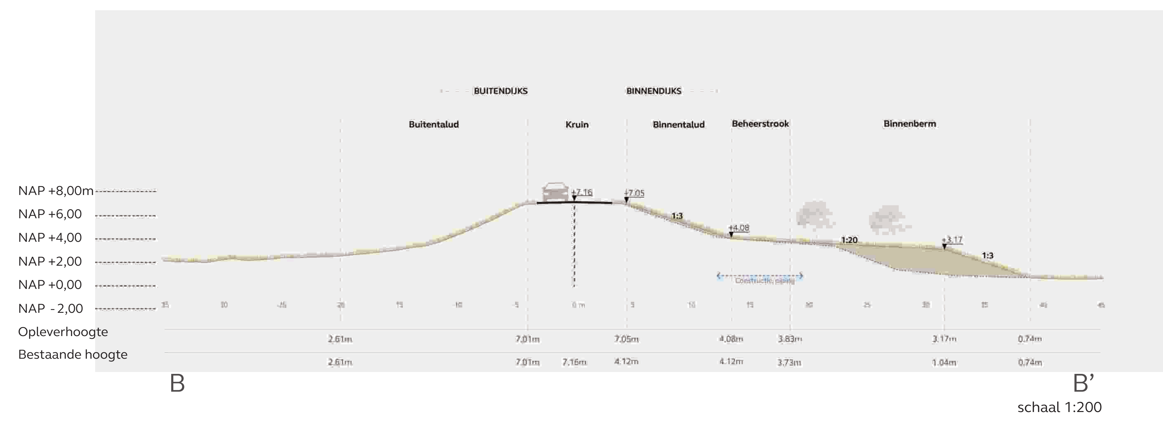
Profiel BB' Verbreding binnenberm
