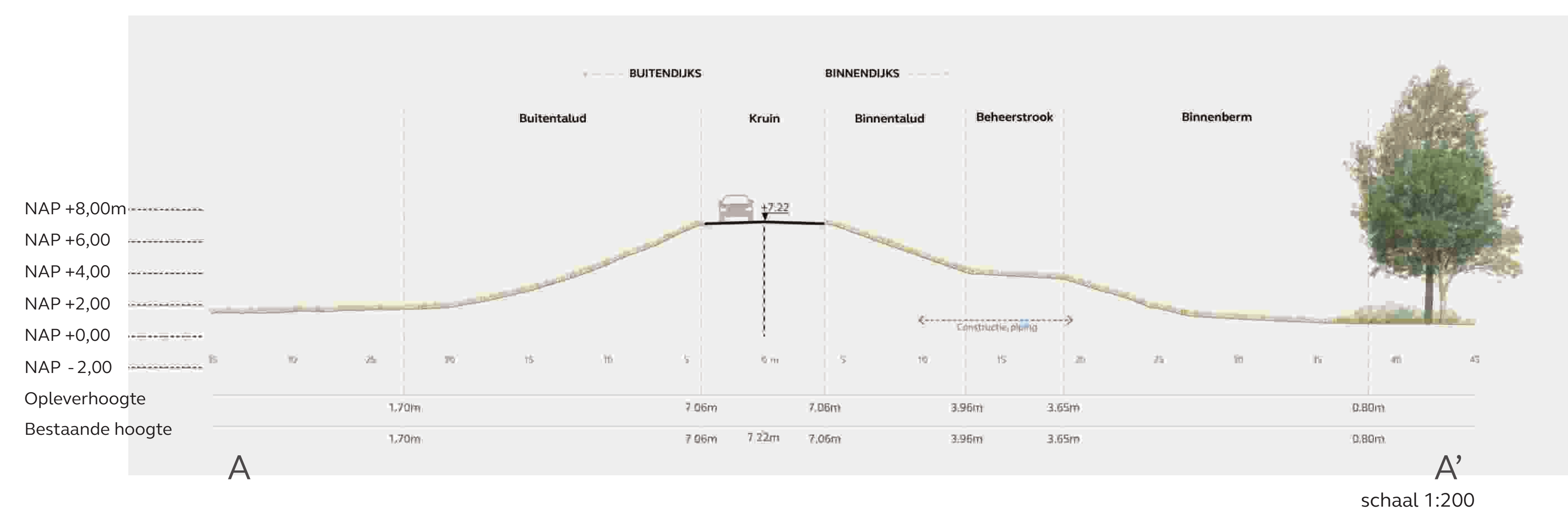
Profiel AA' Filterconstructie in Eendenkooi of constructie piping
