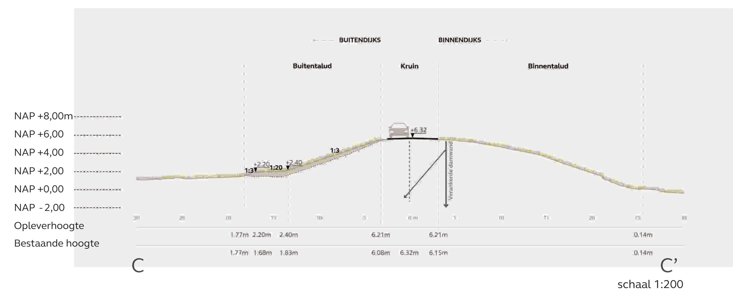
Profiel CC' Buitenwaartse kruinverhoging
