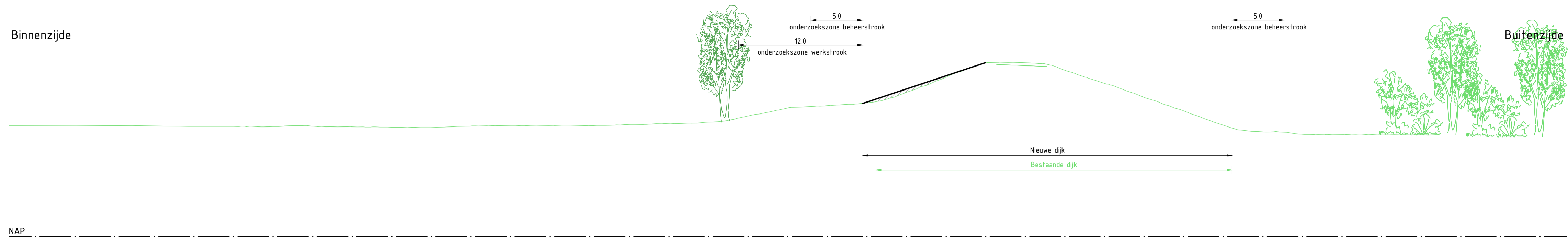
Dwarsprofiel DWP-3a Schaal 1:250
