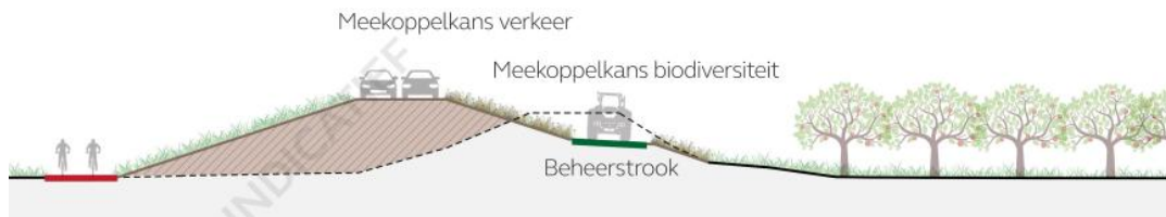
Figuur 13 Alternatief in grond; uitgaande van opgave macrostabiliteit buitendijks (kortere hoge berm)
