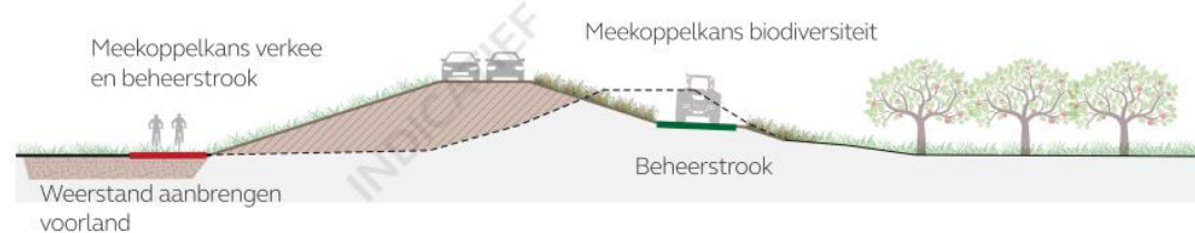
Figuur 14 Alternatief in grond, buitendijks; uitgaande van opgave piping en heave (weerstand voorland), biedt ook oplossing voor macrostabiliteit binnendijks
