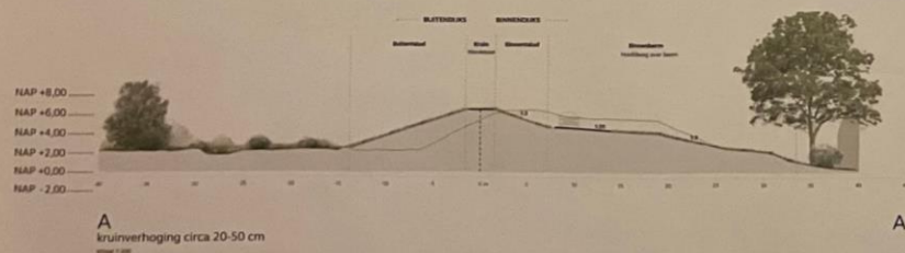
Profiel AA' Buitenwaartse asverschuiving kruinbreedte 3 m
