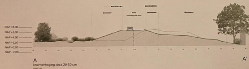
Profiel AA' Buitenwaartse asverschuiving kruinbreedte 9 m
