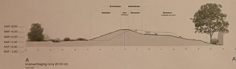
Profiel AA' Buitenwaartse asverschuiving kruinbreedte 3 m
