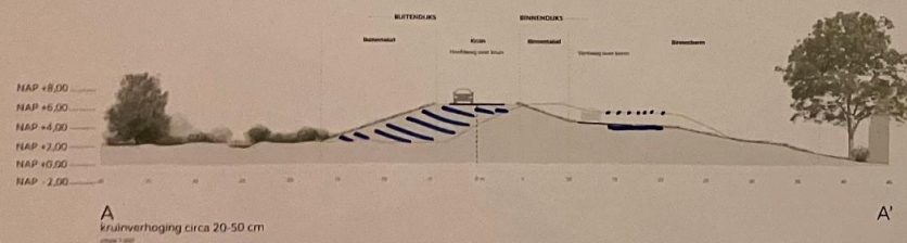
Profiel AA' Buitenwaartse asverschuiving kruinbreedte 9 m
